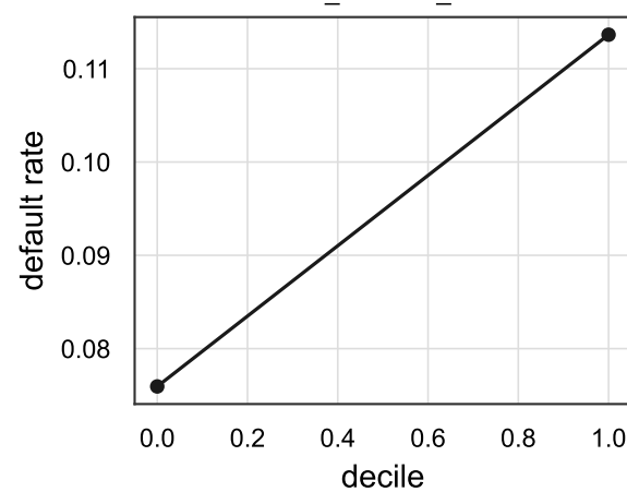
REGION_RATING_CLIENT
