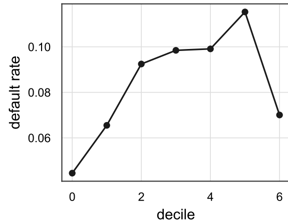
REGION_RATING_CLIENT
