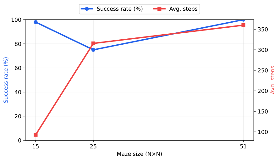
図4 迷路スケール (L3; max steps=250/500/1000) : 成功率 (左軸, 青) と平均ステップ数 (右軸, 赤) のサイズ依存。15 × 15 (max steps=250) と 25 × 25 (max steps=500) では高成功率を保ちつつステップ数を抑え、51 × 51 でもより大きな予算 (max steps=1000) を与えることで成功率を回復できることを示す。
