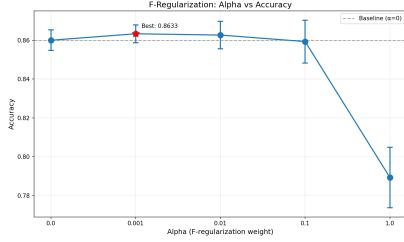
図 6: F 正則化強度 \alpha と SST-2 精度の関係 (DistilBERT, n = 3 seeds, エラーバーは標準偏差). 微弱な正則化 ( \alpha = 0.001 ) で精度が 86.00%→86.33%に改善 ( p = 0.038 ). 過剰な正則化 ( \alpha \geq 0.1 ) は構造を固定化しすぎ性能を悪化させる. この逆 U 字特性は適切な構造化圧の存在を示す.
