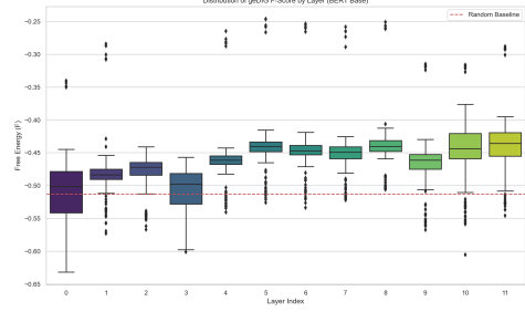
図 5: BERT における層別 \mathcal{F} 値の推移（SST-2, n = 200 文, ヘッド平均）。横軸は層番号、縦軸は \mathcal{F} 値（生の \mathcal{F} ）。破線はランダム行列のベースラインであり、 \mathcal{F} がベースラインより 0 に近い（高い）ほど「ランダムからの構造化」が進む。浅層（Layer 0-1）では \mathcal{F} 値が低く高エントロピーな探索状態にあり、深層（Layer 10-11）では \mathcal{F} 値が上昇し安定した構造化状態に収束する（Layer 0-1 vs 10-11: p < 10^{-80} ）。
