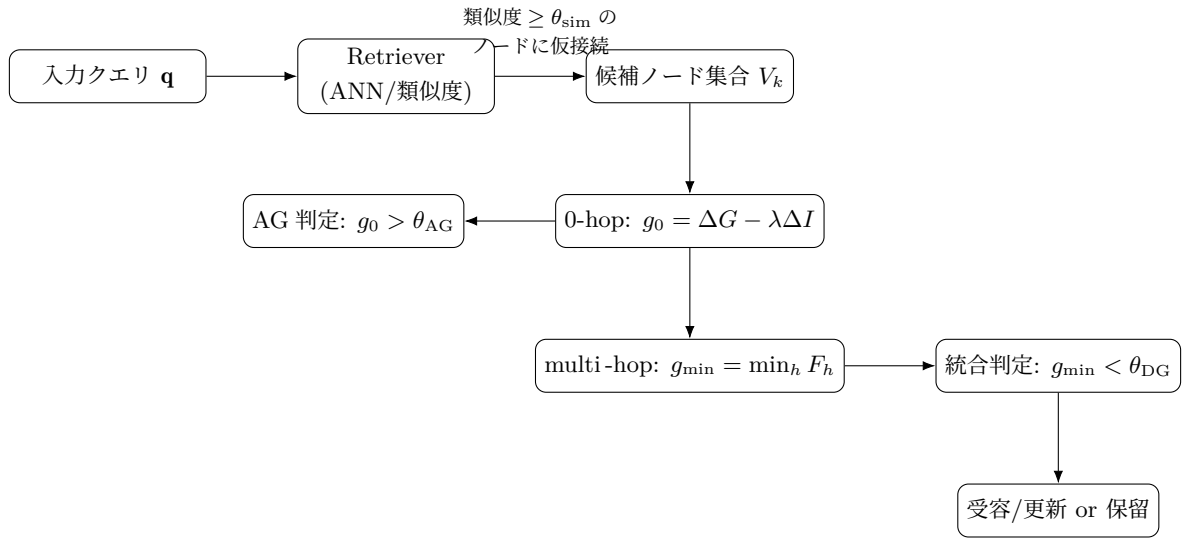
図12 RAG における Phase 1 のワンショット処理フロー。0-hop で曖昧さ（AG）を検知し、条件を満たす場合のみ multi-hop で短絡（経路短縮）を評価し、 g_{\min} < \theta_{\text{DG}} で受容/更新を判断する。
