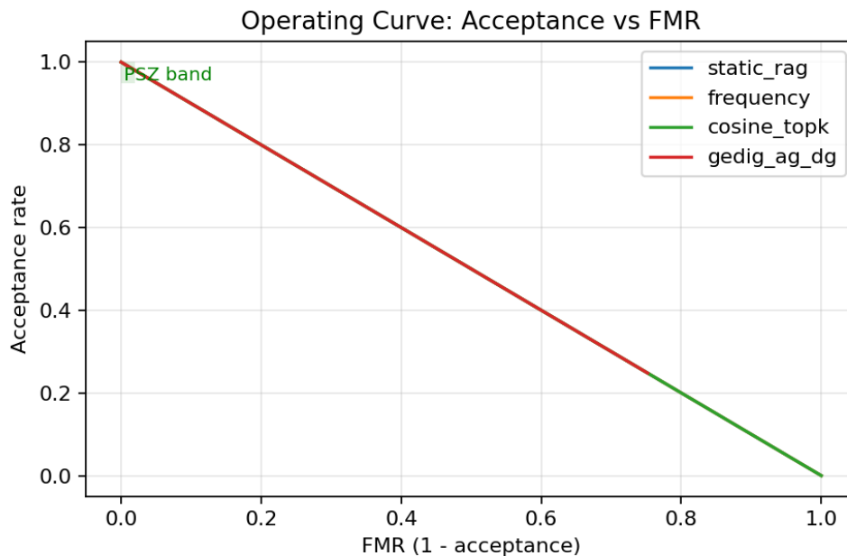
図13 Operating Curves (PSZ 関連；実測)。equal-resources 下での分位掃引により FMR・受容率・遅延のトレードオフを示す（例: p_{AG}=0.92 , p_{DG}=0.08 ；平均 \pm SE, n=16 ）。
