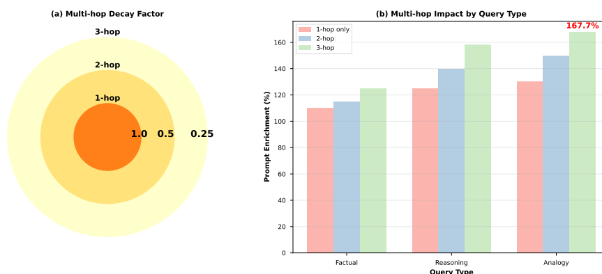
図18 RAG における multi-hop 評価の概念図。H 増加で遠距離の橋が取り込まれ、クロスドメイン推論が促進される。
