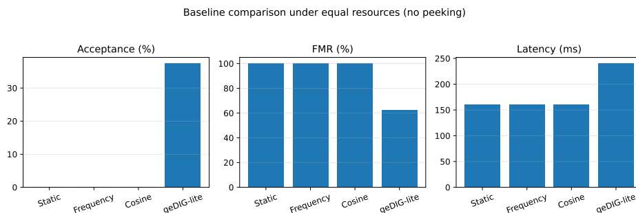
図17 主要指標のベースライン比較 (exp2to4_lite; Static / Frequency / Cosine / geDIG-lite)。geDIG-lite は受容率を押し上げ、追加遅延も同一オーダーに保つ (ただし FMR は高水準に留まる; 本文参照)。
