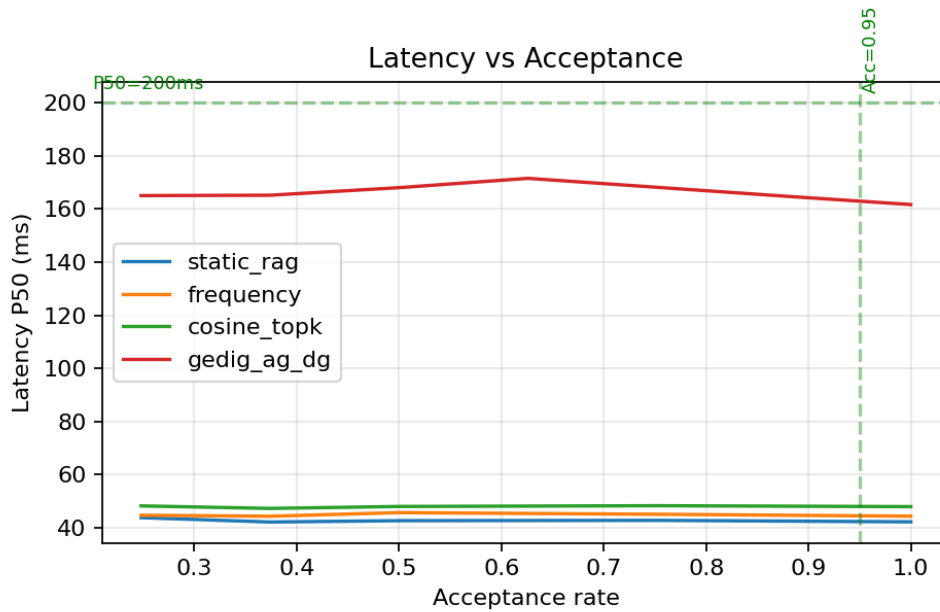
図22 受容率に対する P50 レイテンシ。ガイドライン (Acc=0.95, P50=200ms) を破線で表示。良い方向は P50↓・Acc↑。
