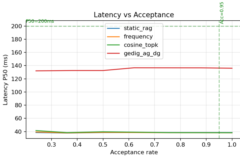
図25 PSZ 目標構成の受容率 vs P50。
