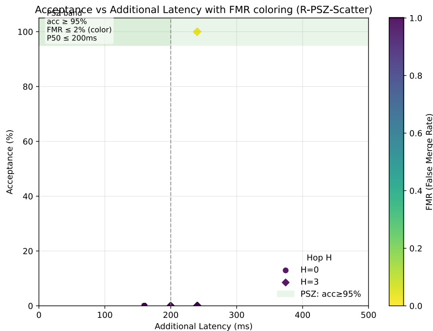
図16 PSZ 分析。各手法の受容率・FMR・追加 P50 遅延を散布図として可視化し、薄緑の帯が PSZ 要件 (受容 \geq 95\% 、FMR \leq 2\% 、P50 \leq 200\text{ms} ) を満たす領域を表す。
