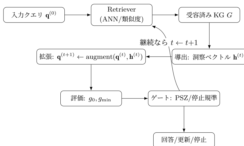
図19 再帰的洞察ベクトルによる段階的強化（RIA）の概念図。各段階で \mathbf{h}^{(t)} を生成しプロンプト/検索を強化、 g_0/g_{\min} の改善と PSZ 制約を満たす限り反復。等価性の主張は行わず、操作的アナロジーとして位置づける。詳細は図12のワンショット版と対比される。
