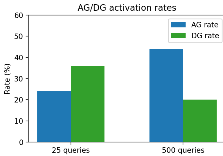
図7 AG/DG 発火率分布（代表例；25 クエリ／ 500 クエリ）。分位制御（ \alpha, \beta ）で設計したターゲット頻度帯に、実測発火率が収まっていることを確認する。
