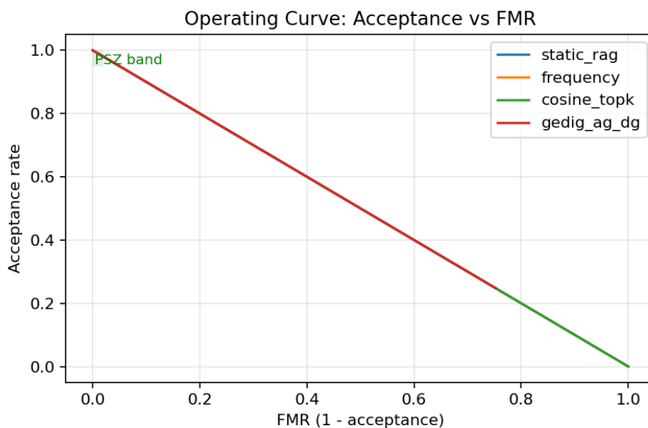
図21 運用曲線 (Acceptance vs FMR)。PSZ 帯 (Acc \geq 0.95, FMR \leq 0.02, P50 \leq 200ms) を重ね描画。良い方向は Acc \uparrow ・FMR \downarrow 。
