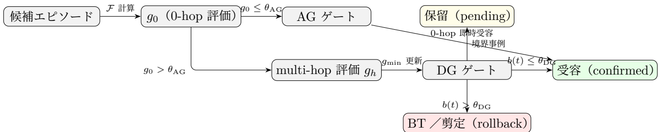
図6 AG/DG フローチャート (概要)。 g_0 (0-hop) で曖昧性検出、 g_{\min} (multi-hop 最小) で洞察確認・受容。バックトラック/剪定は b(t) = \min\{g_0, g_{\min}\} に連動。
