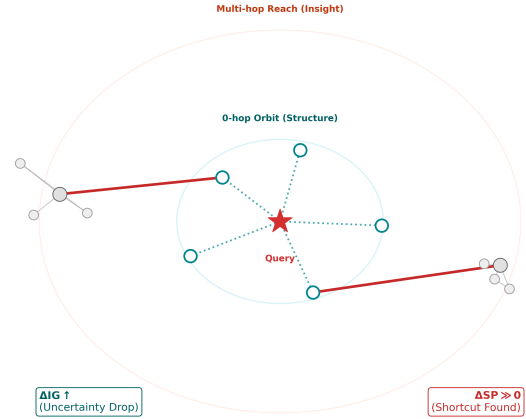
図 1: geDIG による二段階構造化。AG（内側軌道、青）は 0-hop 評価で自由エネルギーが高い状態 ( g_0 > \theta_{\text{AG}} ) を検知し探索を起動する。探索により候補分布が広がると \Delta H > 0 （多様化）が得られ、 \mathcal{F} が低下する。DG（外側軌道、赤）は Multi-hop 評価で経路短縮 ( \Delta\text{SP} > 0 ) を発見し、 g_{\min} < \theta_{\text{DG}} のときエッジを確定する。
