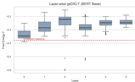
図 5: BERT における層別 F 値の推移 (SST-2, n = 1000 シーケンス平均). 横軸は層番号, 縦軸は F 値 (生の \mathcal{F} ). 破線はランダム行列のベースラインであり, \mathcal{F} がベースラインより 0 に近い (高い) ほど「ランダムからの構造化」が進む. 浅層 (Layer 0-1) では F 値が低く高エントロピーな探索状態にあり, 深層 (Layer 4-5) では F 値が上昇し安定した構造化状態に収束する (Layer 0-1 vs 4-5: p < 0.001 ).
