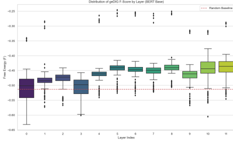
図 5: BERT における層別 F 値の推移 (SST-2, n = 200 文, ヘッド平均). 横軸は層番号, 縦軸は F 値 (生の \mathcal{F} ). 破線はランダム行列のベースラインであり, \mathcal{F} がベースラインより 0 に近い (高い) ほど「ランダムからの構造化」が進む. 浅層 (Layer 0-1) では F 値が低く高エントロピーな探索状態にあり, 深層 (Layer 10-11) では F 値が上昇し安定した構造化状態に収束する (Layer 0-1 vs 10-11: p < 10^{-80} ).
