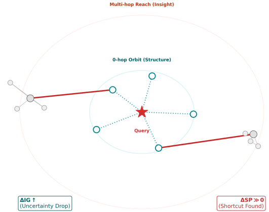
図 1: geDIG による二段階構造化。AG (内側軌道、青) は 0-hop 評価で自由エネルギーが高い状態 ( g_0 > \theta_{\text{AG}} ) を検知し探索を起動する。探索により候補分布が広がると \Delta H > 0 (伸展利得) が得られ、 \mathcal{F} が低下する。DG (外側軌道、赤) は Multi-hop 評価で経路短縮 ( \Delta \text{SP} > 0 ) を発見し、 g_{\text{min}} < \theta_{\text{DG}} のときエッジを確定する。
