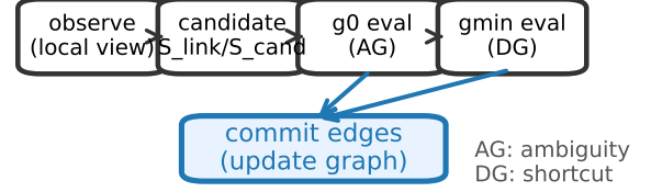
図 2: AG/DG 制御フロー。観測 → 候補生成 → AG 評価 ( g_0 > \theta_{\text{AG}} で探索継続) → DG 評価 ( g_{\text{min}} < \theta_{\text{DG}} でコミット) の事象駆動ループ。AG は局所的異常 (高 \mathcal{F} ) を、DG は大域的効率化 (低 \mathcal{F} ) を検知する。
