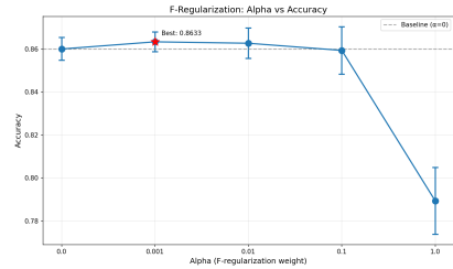
図 6: F 正則化強度 \alpha と SST-2 精度の関係 (DistilBERT, n = 3 seeds, エラーバーは標準偏差). 微弱な正則化 ( \alpha = 0.001 ) で精度が 86.00% \rightarrow 86.33% に改善 ( p = 0.038 ). 過剰な正則化 ( \alpha \geq 0.1 ) は構造を固定化しすぎ性能を悪化させる. この逆 U 字特性は適切な構造化圧の存在を示す.
