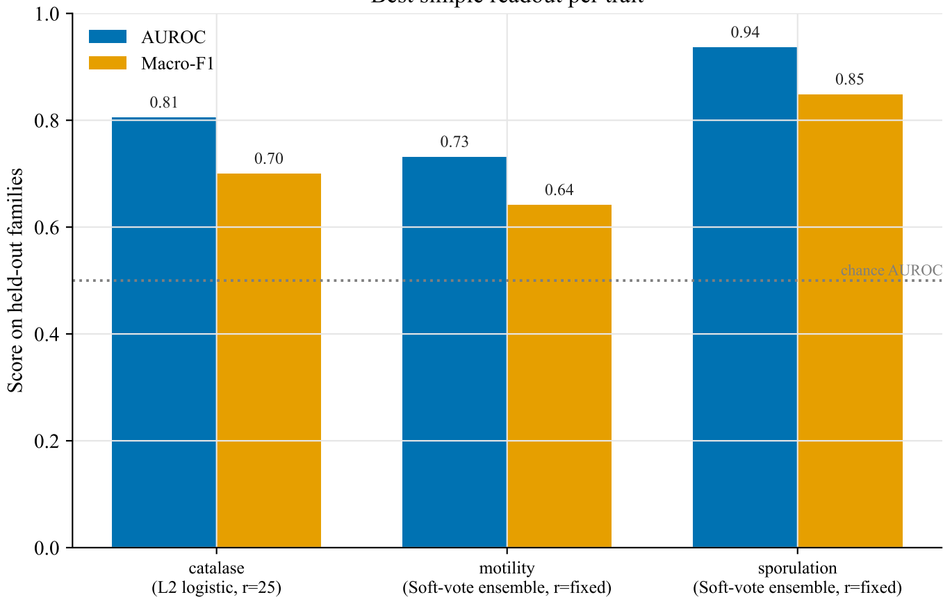
Best simple readout per trait
