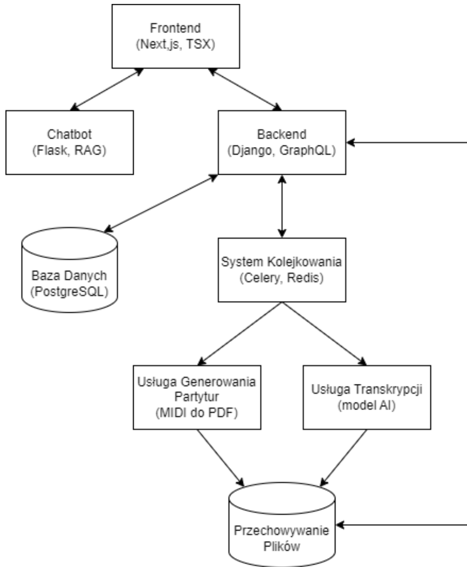
Rysunek 5.1: Diagram architektury systemu TuneScript
