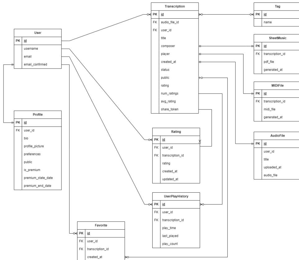
Rysunek 5.2: Schemat bazy danych TuneScript
