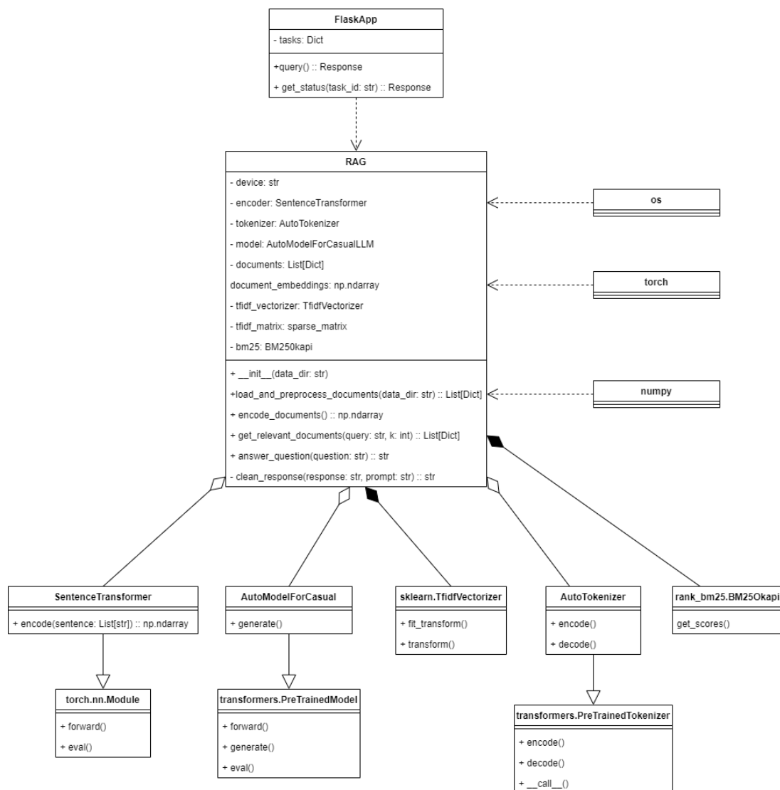
Rysunek 5.3: Diagram klas modułu RAG
