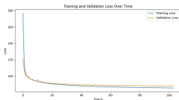
Rysunek: Krzywa uczenia Conditional Convolutional VAE
