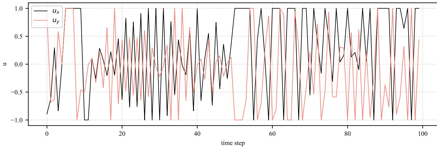
Input trajectory
