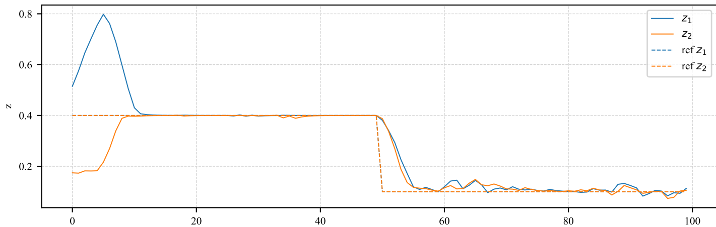
Input trajectory
