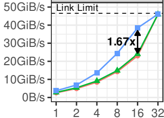
64 KiB Pages
