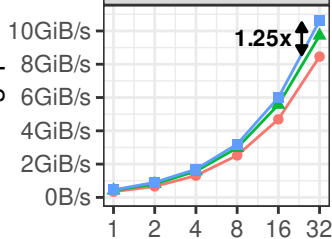
4 KiB Pages
