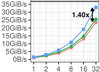
16 KiB Pages
