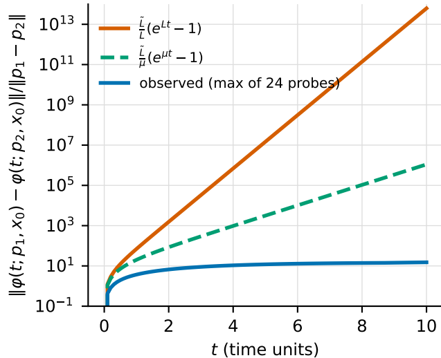
(b) Lemma 2: parameter sensitivity
