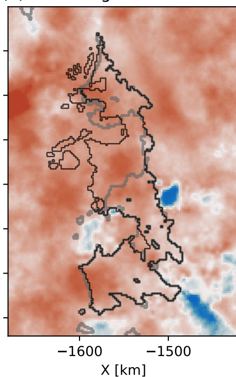
(d) SGS Bouguer realization 2
