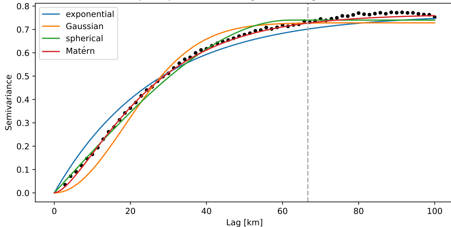
(d) SGS Bouguer realization 2
