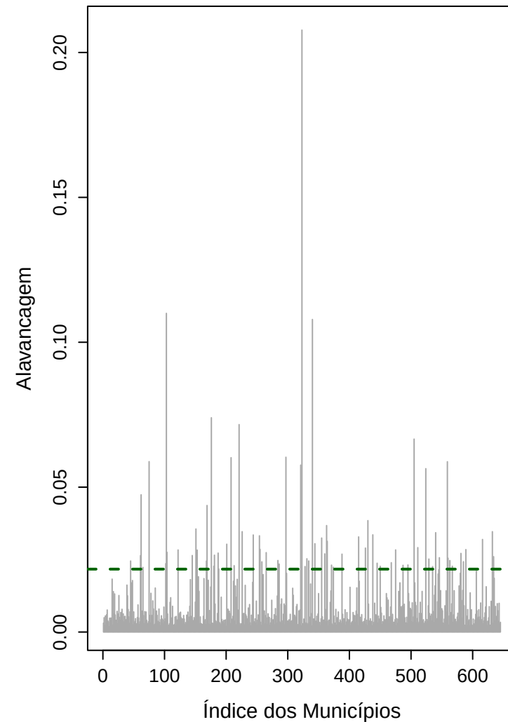
Pontos de Alavanca
