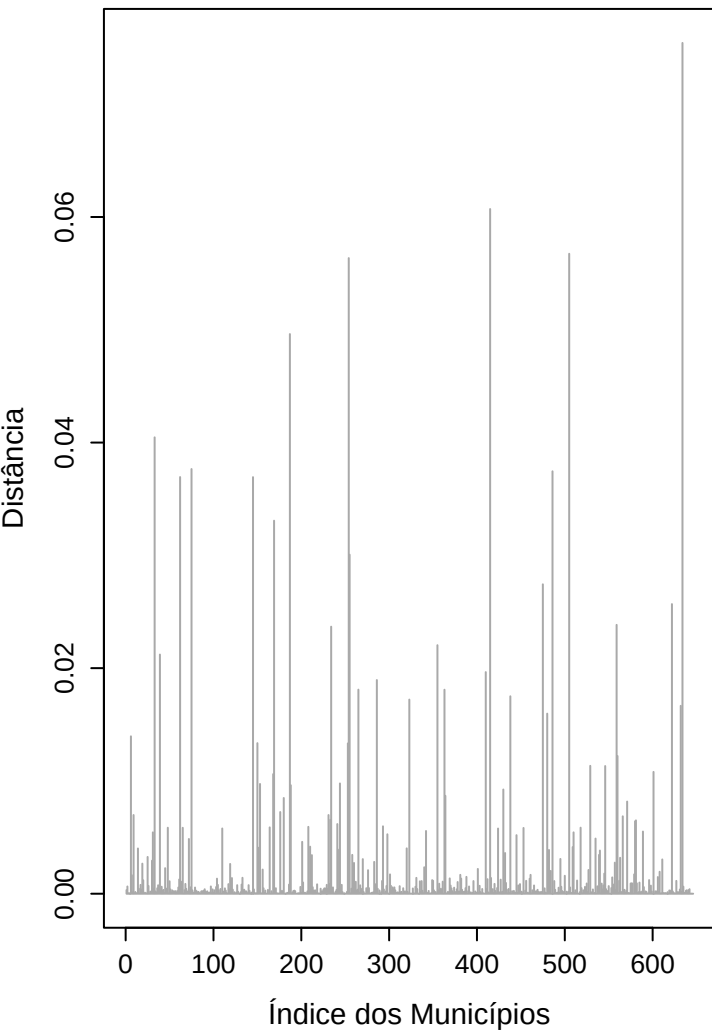
Distância de Cook (Global)
