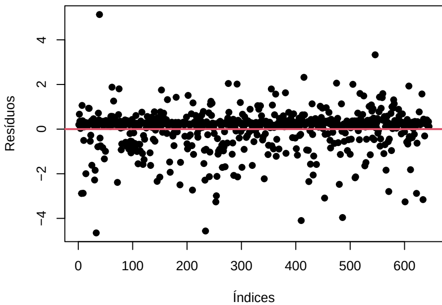
Resíduos Deviance
