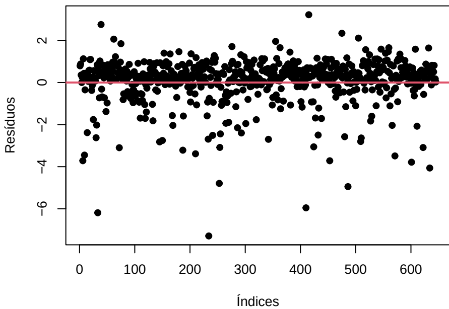
Resíduos Pearson
