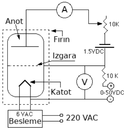
Şekil 1.23: Franck-Hertz deney düzeninin şeması.
