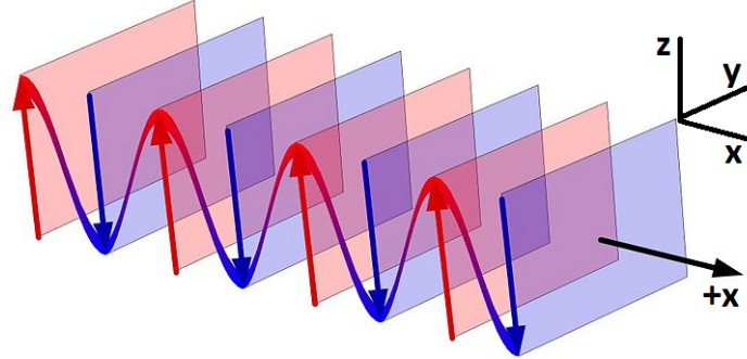
Şekil 2.3: +x yönünde ilerleyen ve y - z düzleminde sabit değerli olan düzlem dalganın temsili çizimi.
