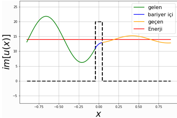
Şekil 4.10: Bir kuantum dalganın sanal kısmının bir bariyer potansiyelinden tünellemesi. Bu örnek için keyfi birimlerde: a = 0.045 , E = 14 , V_0 = 20 ve \hbar = m = 1 alınmıştır. E/V_0 = 14/20 = 0.7 için T > 0.8 olduğu Şekil 4.11'den görülebilir.
