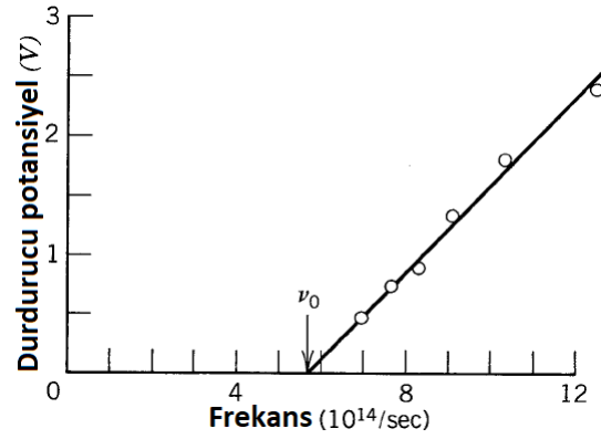
Şekil 1.10: Işık gönderilen plakanın cinsine bağlı olarak belirli bir frekans değerinin altındaki değerlerde fotoelektron koparılamaz [3]. Dolayısıyla \nu_0 frekansının altındaki frekanslar için durdurucu potansiyelin büyüklüğü 0 V'tur.
