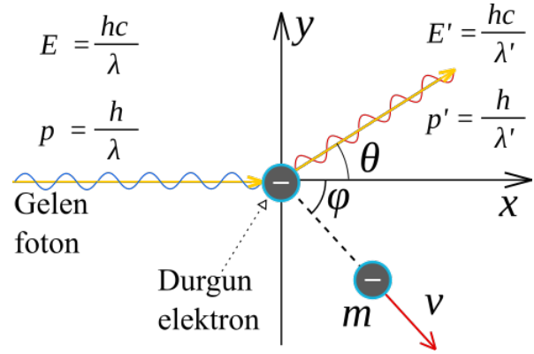
Şekil 1.12: Serbest (veya zayıf bağlı) ve durgun bir elektrona gelen bir fotonun saçılmasının parçacık modeline göre temsili.
