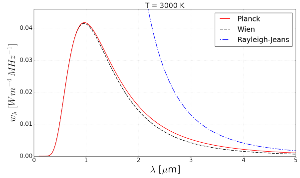
Şekil 1.6: Üç farklı modelle elde edilen kara cisim ışıma spektrumlarının dalga boyuna göre davranışı.
