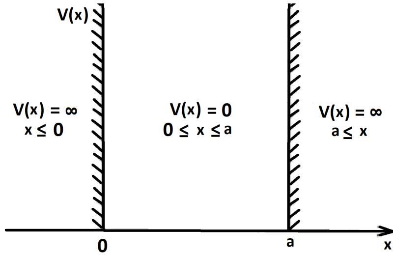
Şekil 3.1: Sonsuz kuyu
