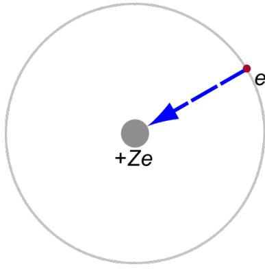
Şekil 1.21: Bohr ve Rutherford atom modeline göre tek elektronlu bir atomik yapının temsili.
