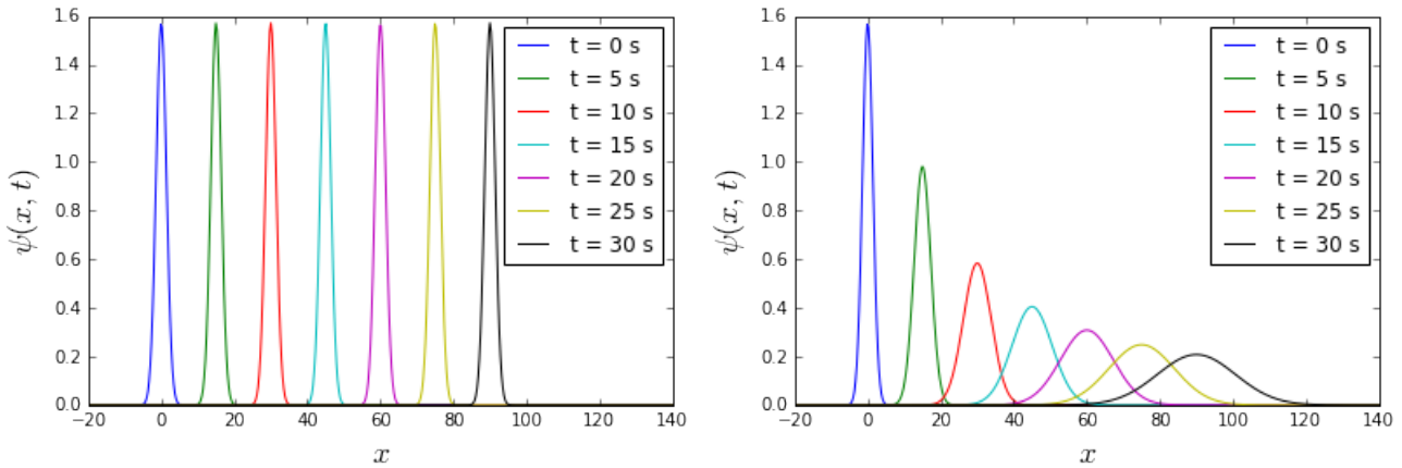
Şekil 2.5: \omega(k)/k sabitken ve k 'nın bir fonksiyonu iken Denk. 2.19 ile hesaplanan |\psi(x, t)|^2 'nin değişimi.
