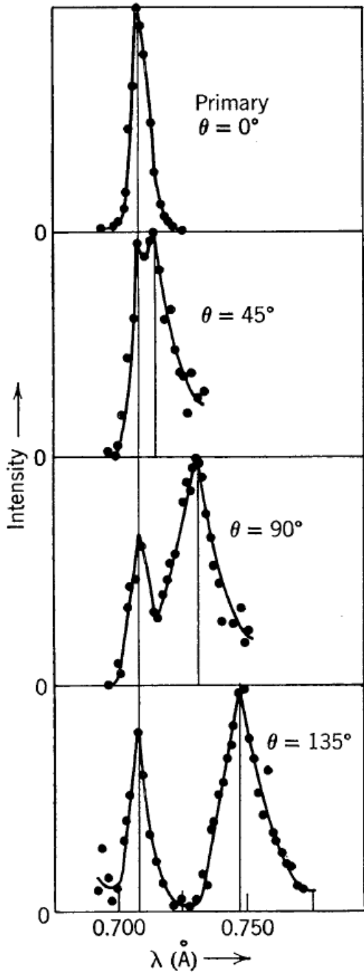
Şekil 1.11: Compton'un deney sonuçları [3, 10, 11]. 0^\circ 'den 135^\circ dereceye kadar çizilen çizgi gelen fotonun (aslında neredeyse kinetik enerji ve momentumunu hiç kaybetmeden saçılan fotonun [11]) dalga boyunu ( \lambda ), diğer çizgiler ise saçılan fotonun dalga boyunu ( \lambda' ) göstermektedir.
