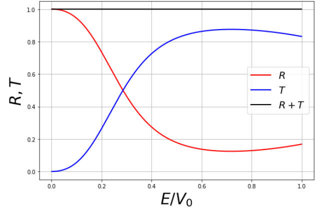
Şekil 4.11: Bu şekilde, Şekil 4.10'daki örnek için, 0 < E/V_0 < 1 aralığında R yansıma ve T geçiş katsayılarının davranışları gösterilmektedir. Klasik fizik açısından yasaklı olan ikinci bölge için geçiş katsayısının sıfır olmadığı açıkça görülmektedir.
