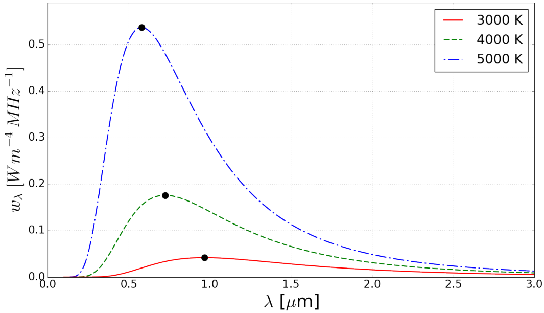
Şekil 1.4: 3000, 4000 ve 5000 Kelvin sıcaklıklarındaki sistemlerin kara cisim spektrumları.
