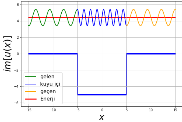
Şekil 4.7: Şekil 4.5'teki E/V_0 = 0.885 değerinde rezonansın varlığı görülebilir. Bu değer için sonlu kuyuda gelen, geçen ve kuyu içindeki dalgaların sanal kısımlarının davranışları görülmektedir.
