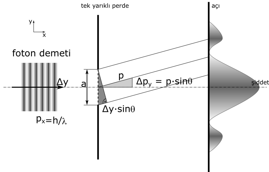
Şekil 2.6: Tek yarıktan geçen ve kırınımına uğrayan foton demeti
