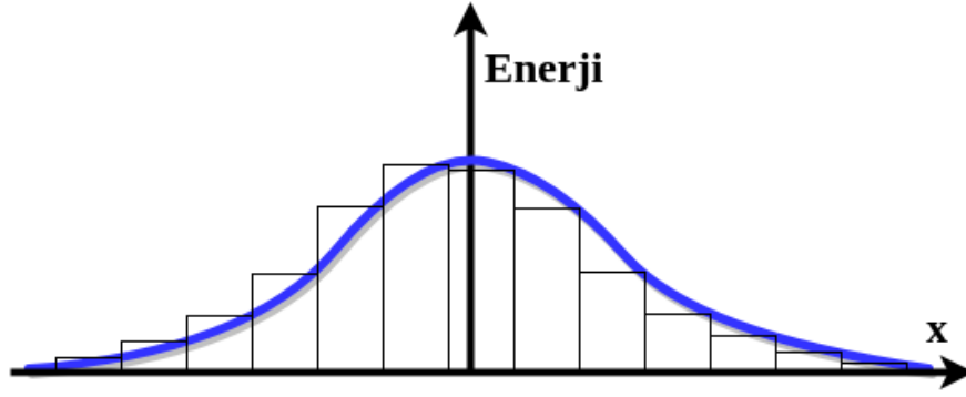
Şekil 4.12: Yavaş değişen bir bariyer potansiyelinin kalın dikdörtgen bariyerler olarak yaklaşık halinin temsili.
