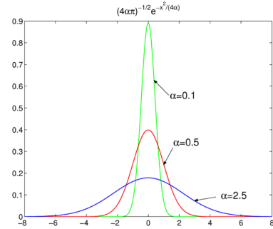
Şekil 3.5: \alpha \rightarrow 0 için Dirac dağılımına yaklaşan bir gaussian fonksiyon.
