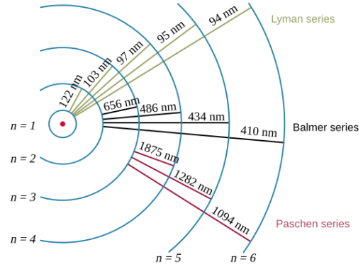
Şekil 1.22: Hidrojen atomu için; elektron geçişleri sırasında yayınlanan fotonların dalga boyları [18].
