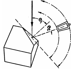
Şekil 1.16: Deneyde kullanılan hedefin geometrik yapısı [15]. Kalın ok gelen elektron demetlerini temsil etmektedir.
