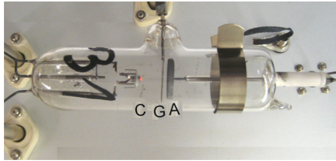
Şekil 1.24: Franck-Hertz deneyinde kullanılan civa dolu tüp. Şekilde Katot (C), Izgara (G) ve Anot (A) işaretlenmiştir.
