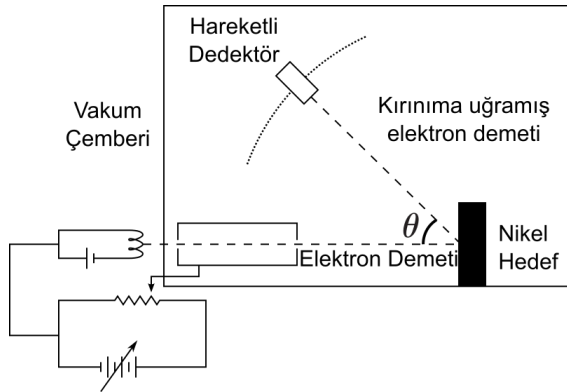
Şekil 1.13: Davisson ve Germer'in deney düzeneğinin şeması[13].
