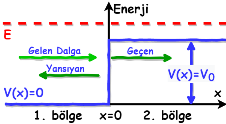
Şekil 4.1: Basamak potansiyeli.
