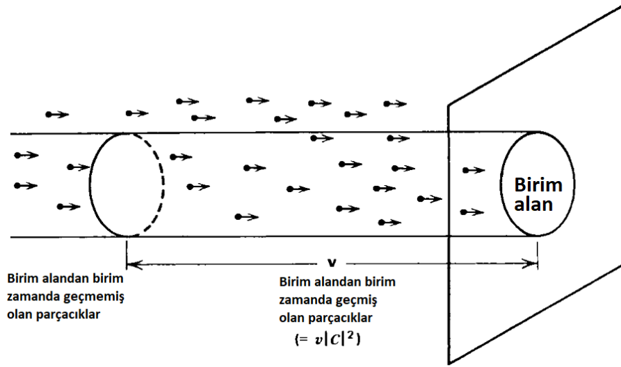
Şekil 3.6: Parçacıkların akısı ve hızları arasındaki bağıntının temsili resmi. Akı: birim zamanda ilgili parçacıkların hızına dik olan birim alandan geçen parçacık sayısıdır.
