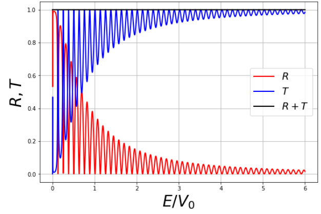
Şekil 4.6: E/V_0 \geq 1 durumunda T \rightarrow 1 ve R \rightarrow 0 davranışlarını göstermektedir. Çünkü enerji arttıkça beklendiği gibi kuyunun yansıma etkisi zayıflamaktadır.
