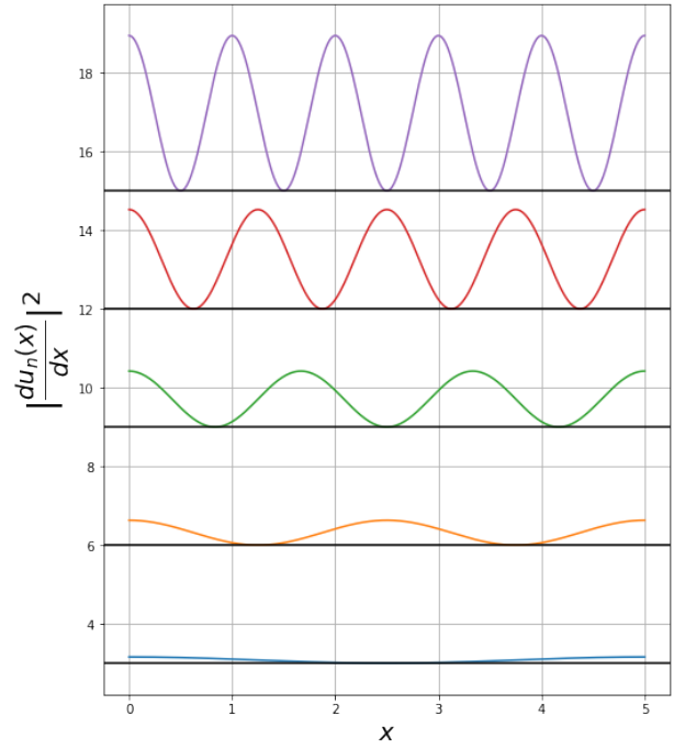
Şekil 3.3: Sonsuz kuyudaki parçacığın özfonksiyonlarının türevlerinin kareleri. Dikkat edilirse artan n ile genlikler de büyümektedir.
