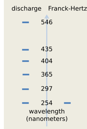
Şekil 1.26: Şeklin sol tarafında civa (Hg) atomlarının uyarılmış atomlarının taban duruma dönebilmek için yayınladıkları fotonların dalga boyu spektrumu verilmiştir. Sağ tarafta ise Franck-Hertz deneyinde gözlenen (254 nm) fotonların dalga boyu verilmiştir.
