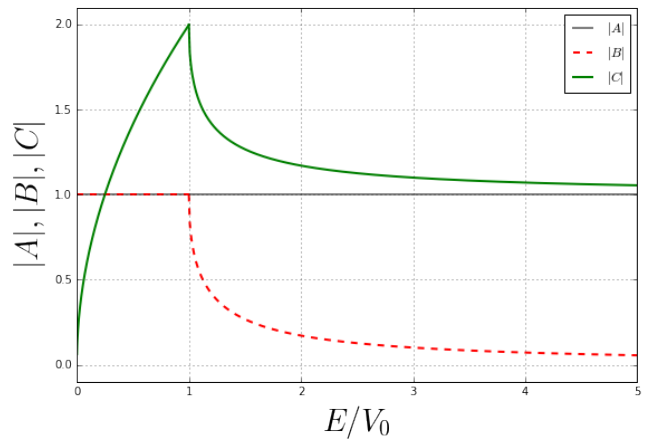
Şekil 4.2: Yansıma ve geçiş katsayılarının E/V_0 'a göre davranışları. Şekil 4.3: Dalga fonksiyonu genliklerinin E/V_0 'a göre davranışları.
