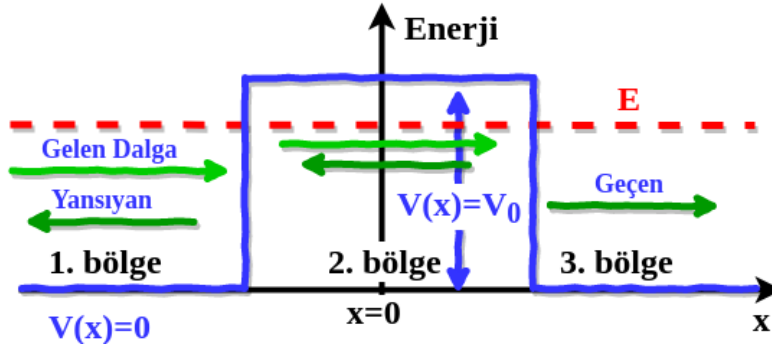
Şekil 4.9: Bariyer potansiyeli, E < V_0 durumu.
