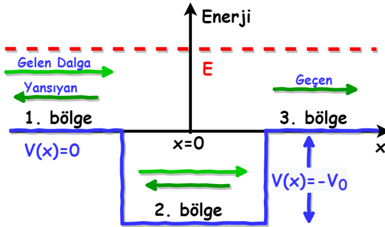
Şekil 4.4: Sonlu kuyu potansiyeli, E > 0 durumu.
