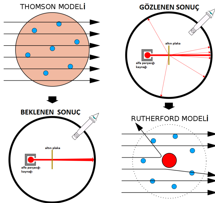
Şekil 1.20: Solda: Thomson tarafından önerilen atom modeli ve bu modele göre alfa saçılım deneyinin beklenen sonucu. Sağda: Gerçekleştirilen deneydeki sonuç ve bu sonuca göre Rutherford'un önerdiği gezegen atom modeli.
