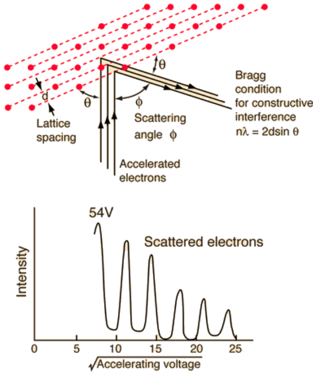
Şekil 1.15: Davisson ve Germer'in deney sonuçları[14].
