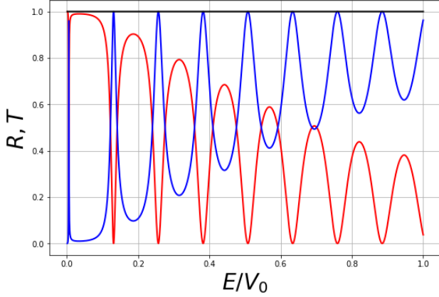
Şekil 4.5: E/V_0 \leq 1 durumunda E \rightarrow 0 oldukça T \rightarrow 0 ve R \rightarrow 1 davranışları göstermelerine karşın, bazı özel enerji değerlerinde ( T = 1 , R = 0 olan yerlerde) "geçiş rezonansları" vardır.
