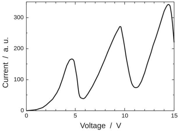
Şekil 1.25: Franck-Hertz deneyinde Katot ve Izgara arasına uygulanan elektrik potansiye-line karşı Anotta oluşan akımın grafiği. Şekildeki çukurlar arası uzaklık 4.9 Volt'tur.
