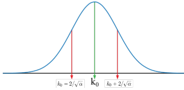
Şekil 2.4: A(k) gaussian dağılım fonksiyonu.
