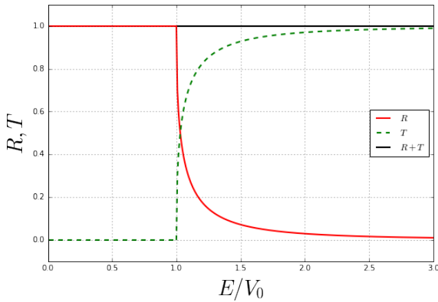
Şekil 4.2: Yansıma ve geçiş katsayılarının E/V_0 'a göre davranışları. Şekil 4.3: Dalga fonksiyonu genliklerinin E/V_0 'a göre davranışları.
