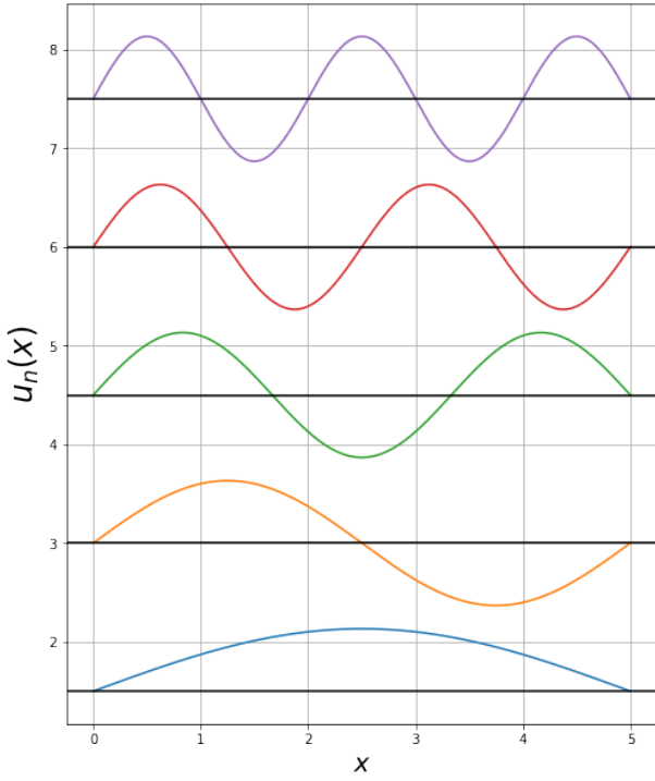
Şekil 3.2: Sonsuz kuyudaki parçacığın özfonksiyonları. Dikkat edilirse genlikler sabit ve artan n değerinden bağımsızdır.
