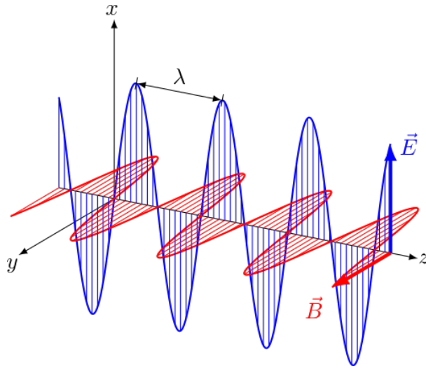
Şekil 1.7: +z yönünde ilerleyen düzlem EM dalgalar.
