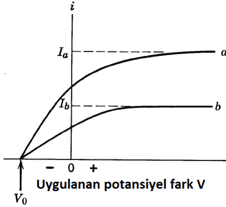
Şekil 1.9: Fotoelektronların (fotoelektrik etkiyle koparılan elektron) sahip olabileceği en büyük kinetik enerjinin ölçümü [3].
