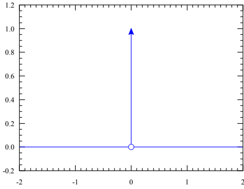
Şekil 3.4: Dirac dağılımı.
