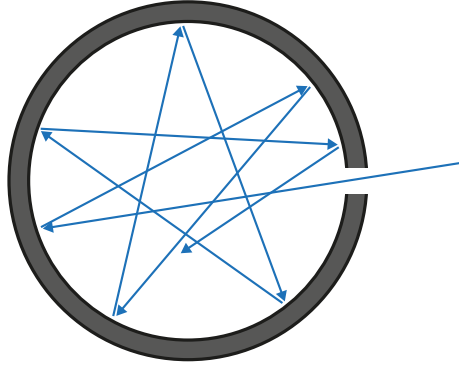
Şekil 1.1: Kara cisim, küre şeklindeki kovukta açılan deliktir.
