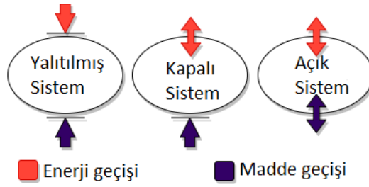
Şekil 1.2: Yalıtılmış, kapalı ve açık sistemlerin temsili.
