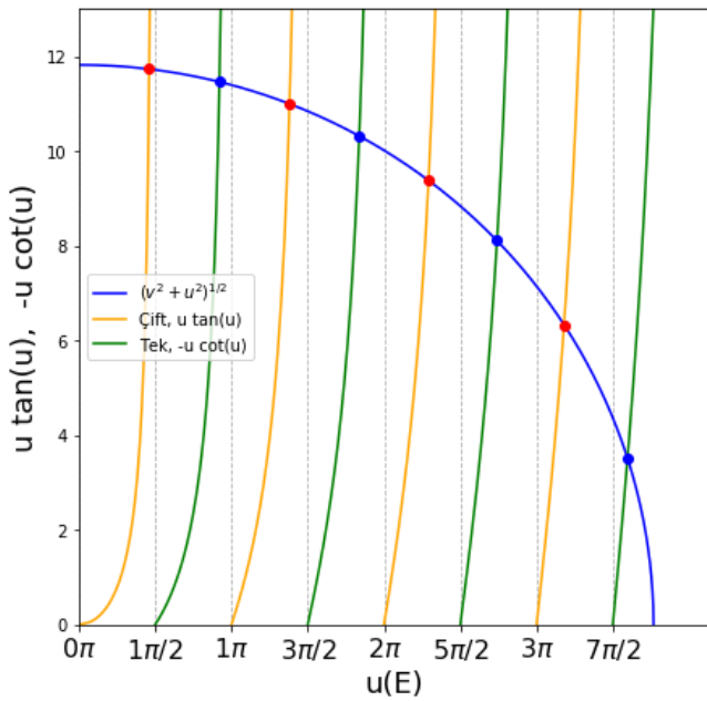
Şekil 4.14: Transandantal denklemlerin tek ve çift çözümleri.
