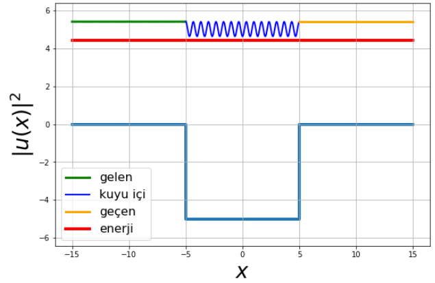
Şekil 4.8: Şekil 4.5'teki E/V_0 = 0.885 değerinde rezonansın varlığı görülebilir. Bu değer için sonlu kuyuda gelen, geçen ve kuyu içindeki dalgaların karelerinin (olasılık yoğunluklarının) davranışları görülmektedir.
