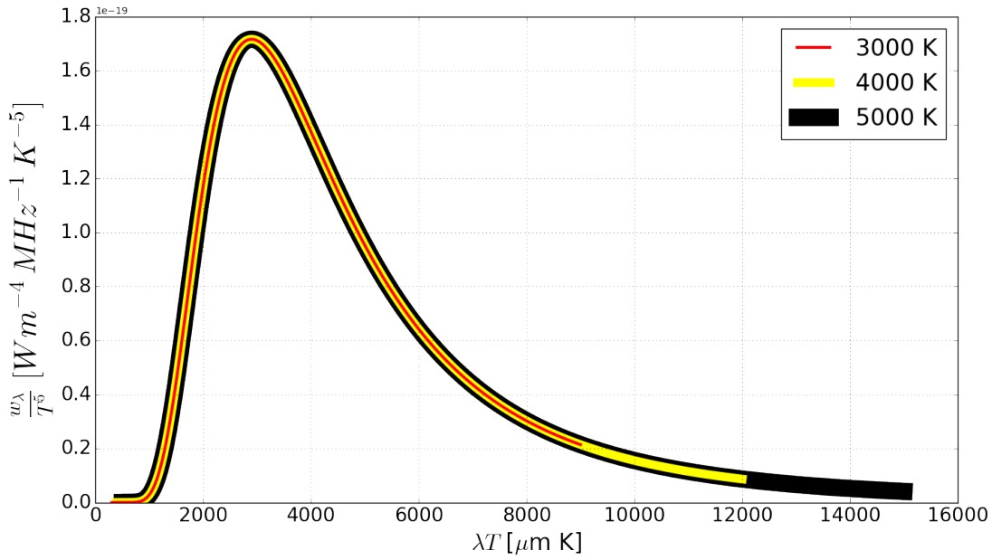
Şekil 1.3: Denk. 1.2'deki fonksiyonun varlığını gösteren spektrum.
