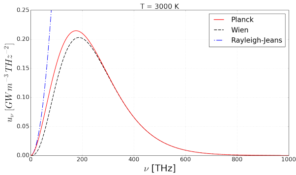
Şekil 1.5: Üç farklı modelle elde edilen kara cisim ışıma spektrumlarının frekansa göre davranışı.
