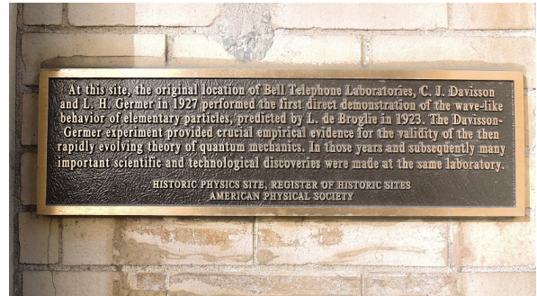
Şekil 1.13: Davisson ve Germer'in anısına düzenlenen deneyin gerçekleştirildiği Bell laboratuvarındaki anı tablosu[13].
