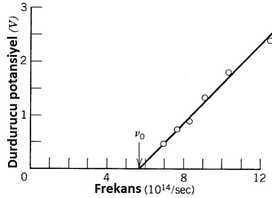
Şekil 1.10: Işık gönderilen plakanın cinsine bağlı olarak belirli bir frekans değerinin altındaki değerlerde fotoelektron koparılmaz [3]. Dolayısıyla \nu_0 frekansının altındaki frekanslar için durdurucu potansiyelin büyüklüğü 0 V'tur.
