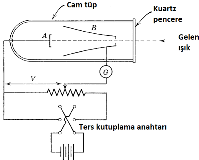
Şekil 1.8: Hertz tarafından kullanılan deney düzeneğinin şeması [3].
