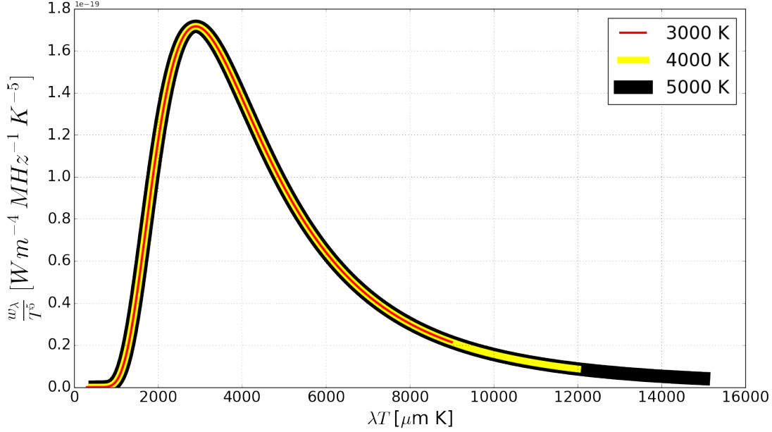
Şekil 1.3: Denk. 1.4'deki fonksiyonun varlığını gösteren spektrum.
