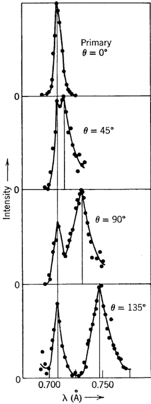
Şekil 1.11: Compton'un deney sonuçları [10, 3, 11]. 0^\circ 'den 135^\circ dereceye kadar çizilen çizgi gelen fotonun (aslında neredeyse kinetik enerji ve momentumunu hiç kaybetmeden saçılan fotonun [11]) dalga boyunu ( \lambda ), diğer çizgiler ise saçılan fotonun dalga boyunu ( \lambda' ) göstermektedir.
