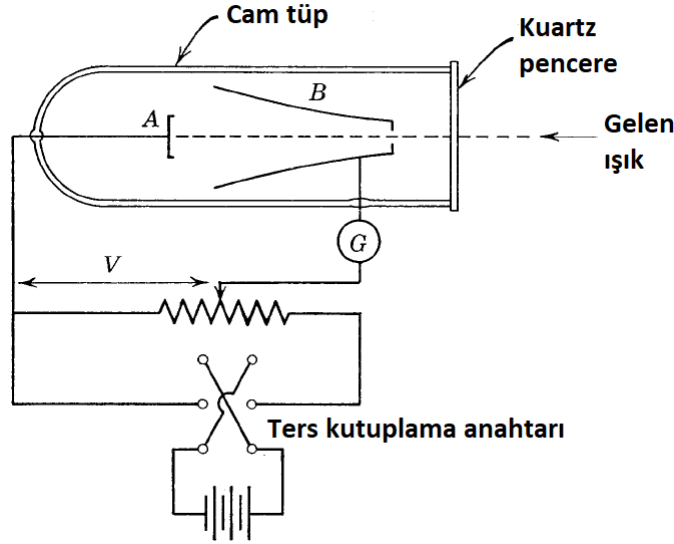
Şekil 1.8: Hertz tarafından kullanılan deney düzeni [3].
