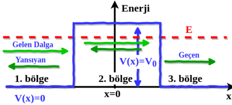
Şekil 9: Bariyer potansiyeli, E < V_0 durumu.
