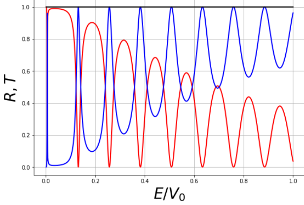
Şekil 5: E/V_0 \leq 1 durumunda E \rightarrow 0 oldukça T \rightarrow 0 ve R \rightarrow 1 davranışları göstermelerine karşın, bazı özel enerji değerlerinde ( T = 1, R = 0 olan yerlerde) “geçiş rezonansları” vardır.
