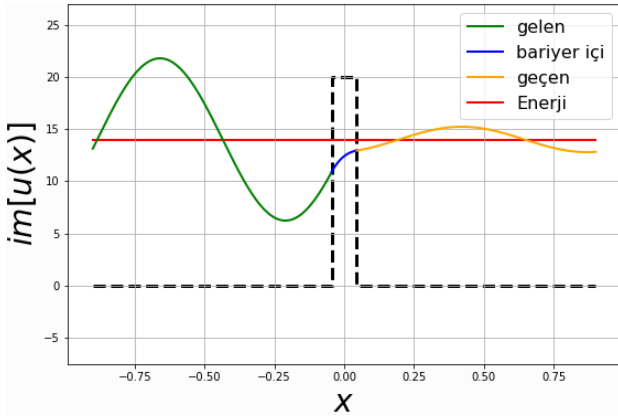
Şekil 10: Bir kuantum dalganın sanal kısmının bir bariyer potansiyelinden tünellemesi. Bu örnek için keyfi birimlerde: a = 0.045 , E = 14 , V_0 = 20 ve \hbar = m = 1 alınmıştır. E/V_0 = 14/20 = 0.7 için T > 0.8 olduğu Şekil 11'den görülebilir.
