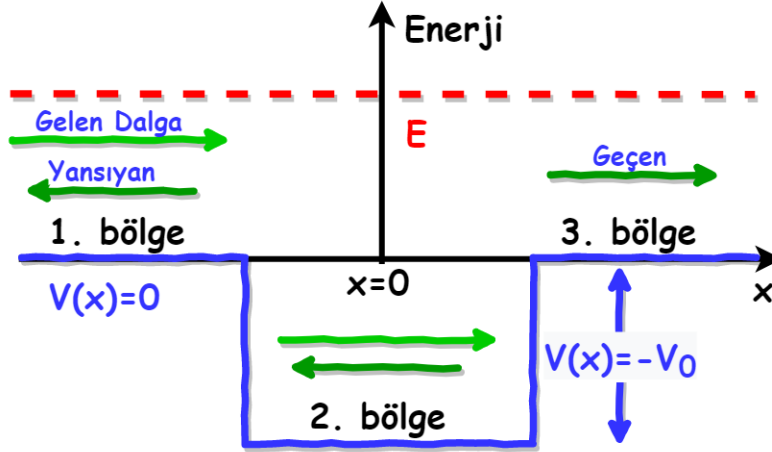
Şekil 4: Sonlu kuyu potansiyeli, E > 0 durumu.
