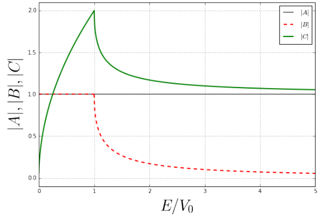
Şekil 2: Yansıma ve geçiş katsayılarının E/V_0 'a göre davranışları. Şekil 3: Dalga fonksiyonu genliklerinin E/V_0 'a göre davranışları.
