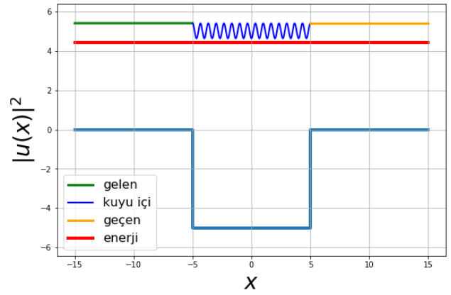
Şekil 8: Şekil 5’teki E/V_0 = 0.885 değerinde rezonansın varlığı görülebilir. Bu değer için sonlu kuyuda gelen, geçen ve kuyu içindeki dalgaların karelerinin (olasılık yoğunluklarının) davranışları görülmektedir.
