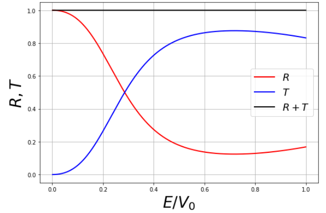
Şekil 11: Bu şekilde, Şekil 10'daki örnek için, 0 < E/V_0 < 1 aralığında R yansıma ve T geçiş katsayılarının davranışları gösterilmektedir. Klasik fizik açısından yasaklı olan ikinci bölge için geçiş katsayısının sıfır olmadığı açıkça görülmektedir.
