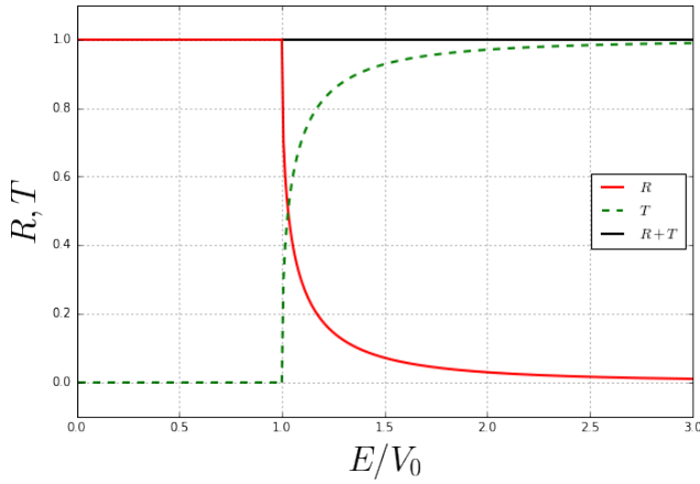
Şekil 2: Yansıma ve geçiş katsayılarının E/V_0 'a göre davranışları. Şekil 3: Dalga fonksiyonu genliklerinin E/V_0 'a göre davranışları.
