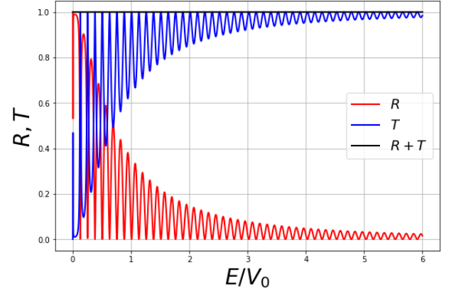
Şekil 6: E/V_0 \geq 1 durumunda T \rightarrow 1 ve R \rightarrow 0 davranışlarını göstermektedir. Çünkü enerji arttıkça beklediği gibi kuyunun yansıtma etkisi zayıflamaktadır.
