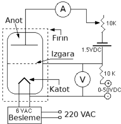
Şekil 23: Franck-Hertz deney düzenine şeması.
