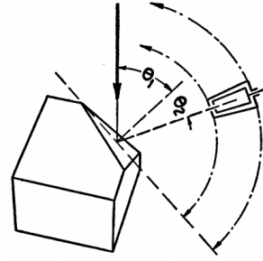
Şekil 16: Deneyde kullanılan hedefin geometrik yapısı [7]. Kalın ok gelen elektron demetlerini temsil etmektedir.
