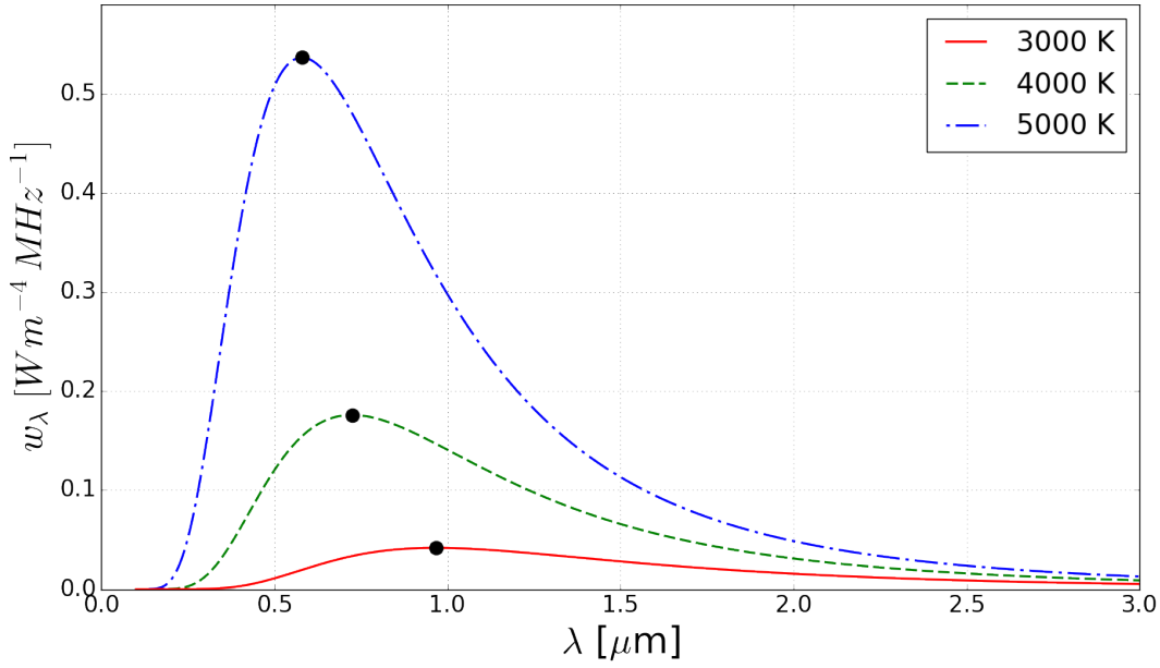
Şekil 4: 3000, 4000 ve 5000 Kelvin sıcaklıklarındaki sistemlerin kara cisim spektrumları.
