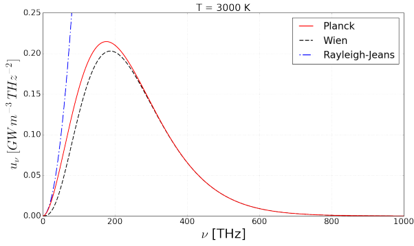
Şekil 5: Üç farklı modelle elde edilen kara cisim ışıma spektrumlarının frekansa göre davranışı.
