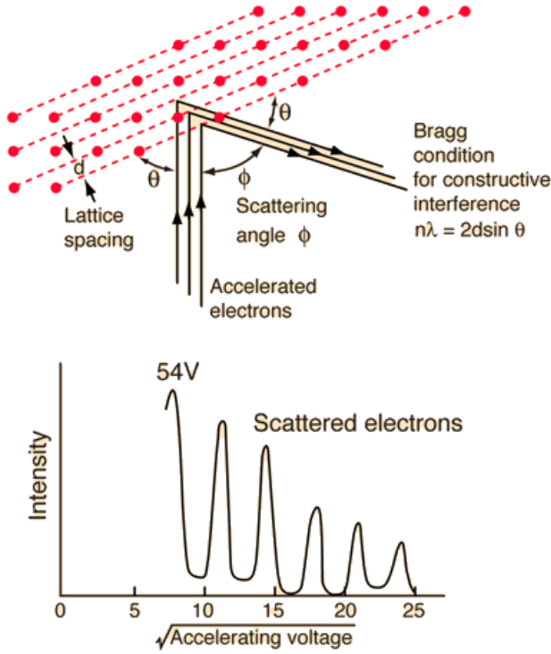
Şekil 15: Davisson ve Germer'in deney sonuçları[12].
