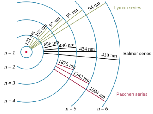
Şekil 22: Hidrojen atomu için; elektron geçişleri sırasında yayımlanan fotonların dalga boyları [6].
