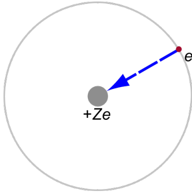
Şekil 21: Bohr ve Rutherford atom modeline göre tek elektronlu bir atomik yapının temsili.
