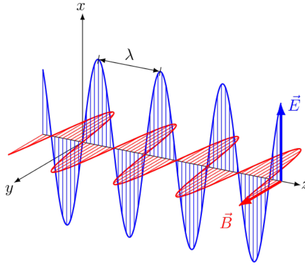
Şekil 7: +z yönünde ilerleyen düzlem EM dalgalar.
