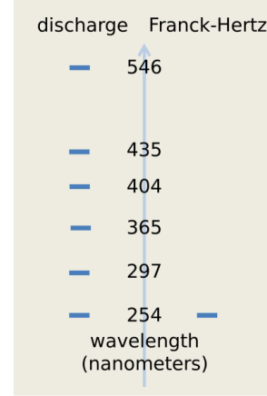
Şekil 26: Şeklin sol tarafında civa (Hg) atomlarının uyarılmış atomlarının taban duruma dönebilmek için yayınladıkları fotonların dalga boyu spektrumu verilmiştir. Sağ tarafta ise Franck-Hertz deneyinde gözlenen (254 nm) fotonların dalga boyu verilmiştir.
