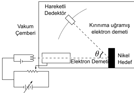
Şekil 13: Davisson ve Germer'in deney düzeneğinin şeması[4].
