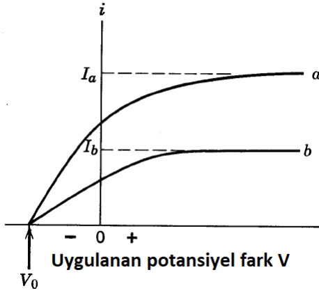
Şekil 9: Fotoelektronların (fotoelektrik etkiyle koparılan elektron) sahip olabileceği en büyük kinetik enerjinin ölçümü [8].
