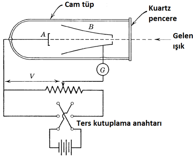
Şekil 8: Hertz tarafından kullanılan deney düzeneğinin şeması [8].
