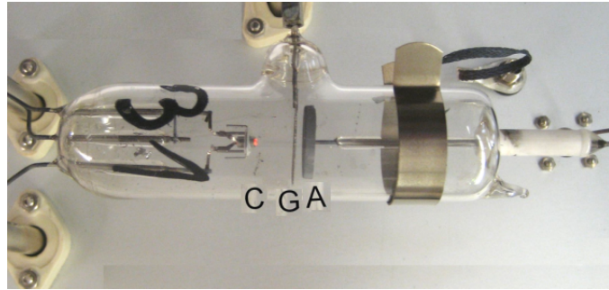
Şekil 24: Franck-Hertz deneyinde kullanılan civa dolu tüp. Şekilde Katot (C), Izgara (G) ve Anot (A) işaretlenmiştir.
