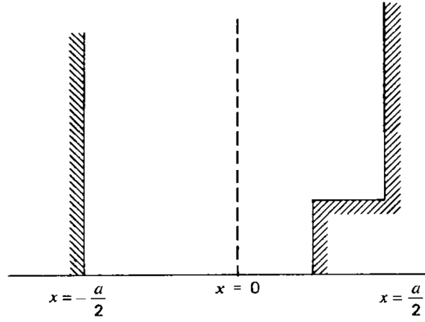
Şekil 7: Yansıma (ayna) simetrisi içermeyen bir potansiyel örneği.
