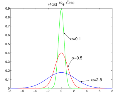
Şekil 5: \alpha \rightarrow 0 için Dirac dağılımına yaklaşan bir gausyen fonksiyon.
