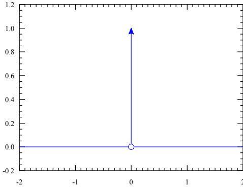
Şekil 4: Dirac dağılımı.
