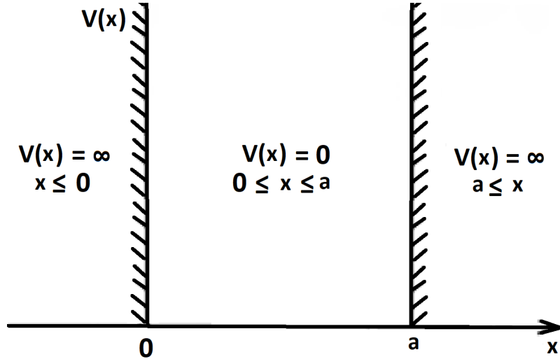
Şekil 1: Sonsuz kuyu
