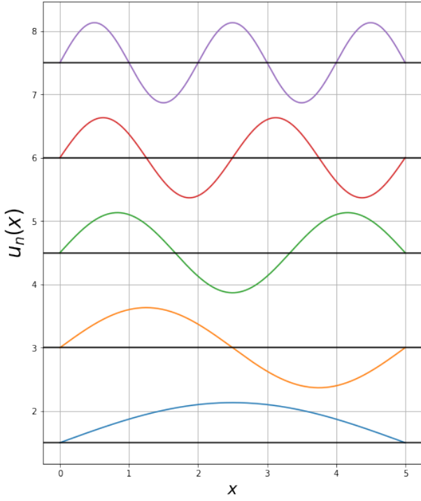
Şekil 2: Sonsuz kuyudaki parçacığın özfonksiyonları. Dikkat edilirse genlikler sabit ve artan n değerinden bağımsızdır.
