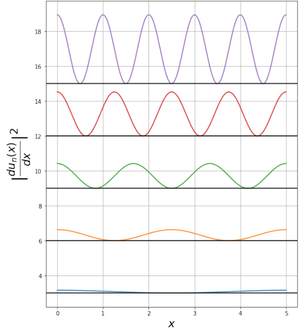
Şekil 3: Sonsuz kuyudaki parçacığın özfonksiyonlarının türevlerinin kareleri. Dikkat edilirse artan n ile genlikler de büyümektedir.
