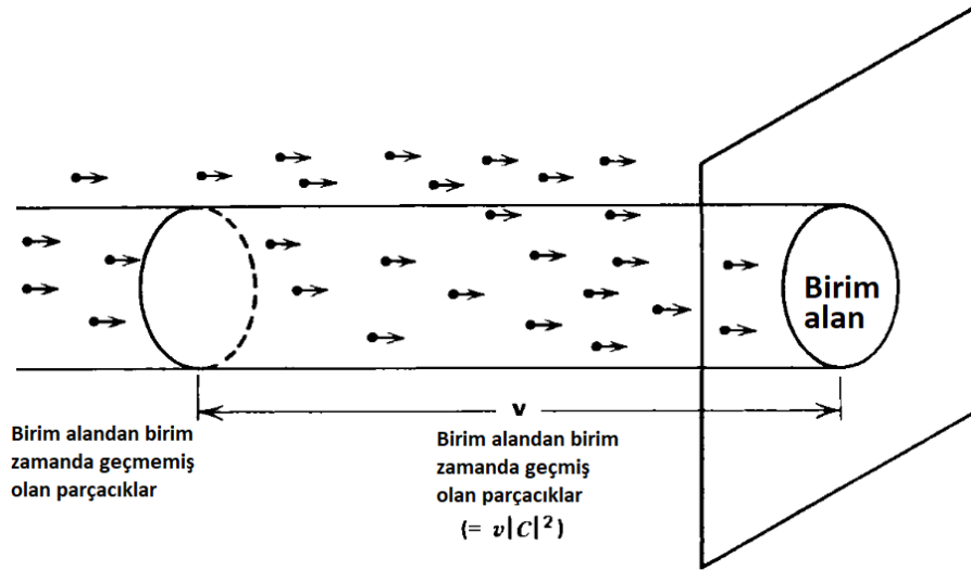
Şekil 6: Parçacıkların akısı ve hızları arasındaki bağıntının temsili resmi. Akı: birim zamanda ilgili parçacıkların hızına dik olan birim alandan geçen parçacık sayısıdır.
