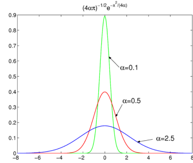
Şekil 3.5: \alpha \rightarrow 0 için Dirac dağılımına yaklaşan bir gaussian fonksiyon.
