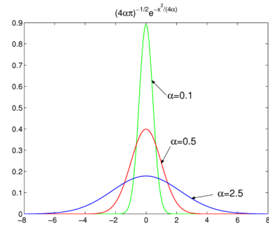
Şekil 3.5: \alpha \rightarrow 0 için Dirac dağılımına yaklaşan bir gausyen fonksiyon.
