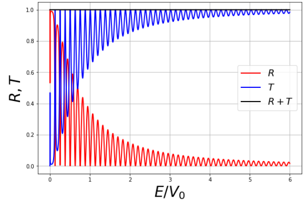
Şekil 4.6: E/V_0 \geq 1 durumunda T \rightarrow 1 ve R \rightarrow 0 davranışlarını göstermektedir. Çünkü enerji arttıkça beklendiği gibi kuyunun yansıtma etkisi zayıflamaktadır.
