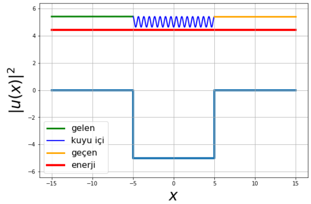
Şekil 4.8: Şekil 4.5'teki E/V_0 = 0.885 değerinde rezonansın varlığı görülebilir. Bu değer için sonlu kuyuda gelen, geçen ve kuyu içindeki dalgaların karelerinin (olasılık yoğunluklarının) davranışları görülmektedir.
