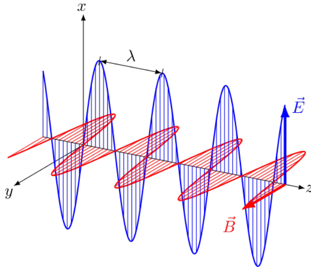
Şekil 1.6: +z yönünde ilerleyen düzlem EM dalgalar.
