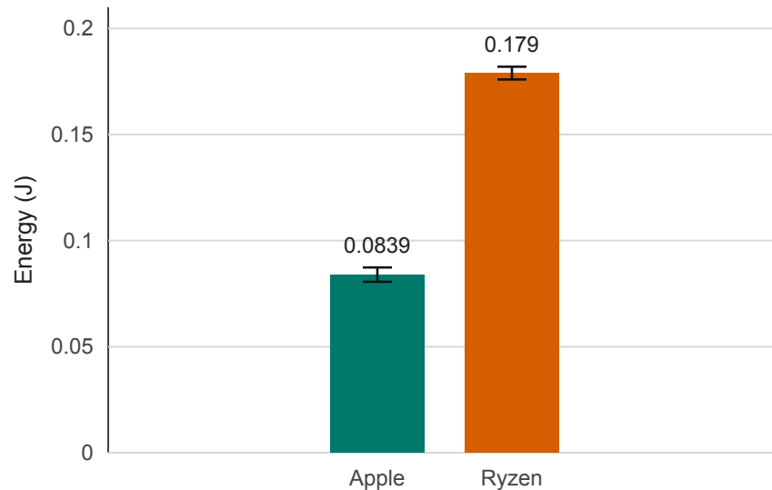
matmul 256x256
