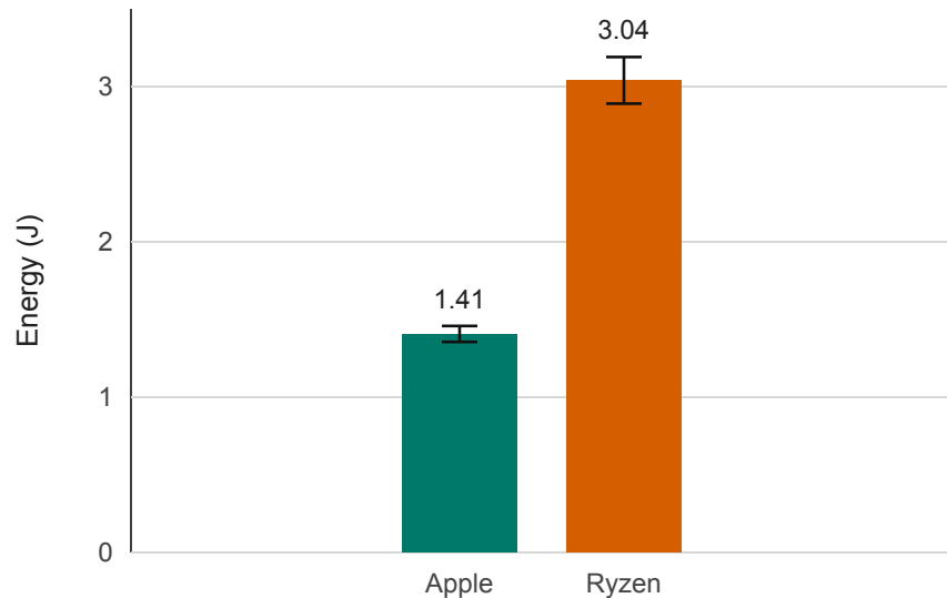
fib(40)
