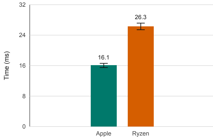
matmul 256x256
