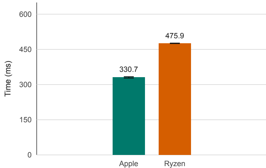
fib(40)
