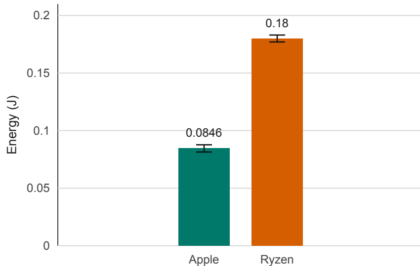
matmul 256x256
