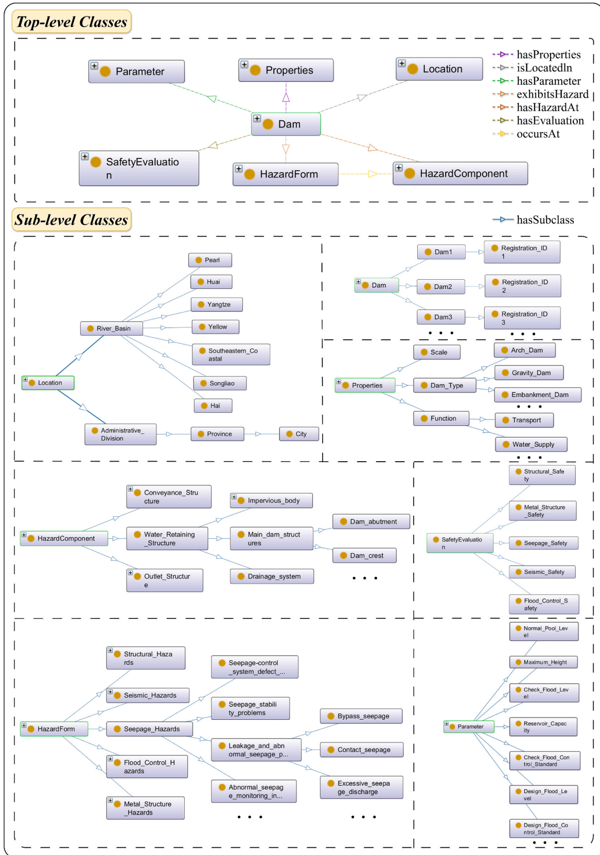
Fig. 2. DDO in Protégé.
