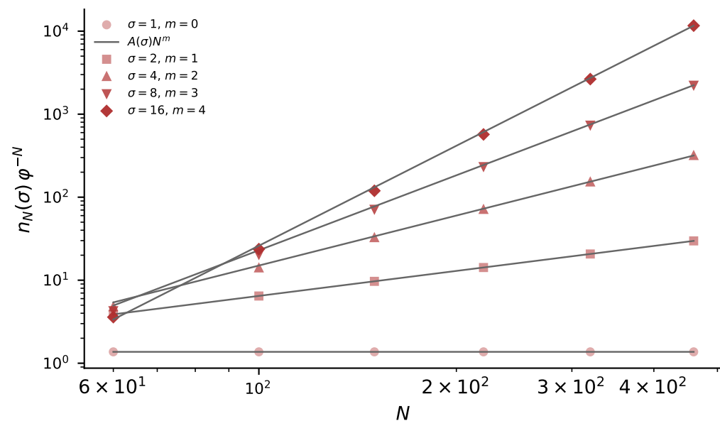
(d) W_{108}/W_{201} : n_N(\sigma) \approx A(\sigma)N^m\varphi^N
