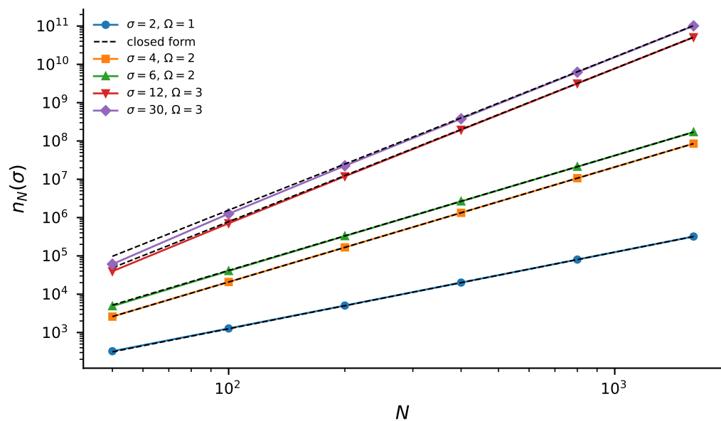
(c) W_{156}/W_{198} : n_N(\sigma) \approx P(\sigma)(N/2)^{\Omega+1}/(\Omega+1)!
