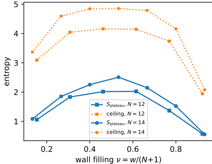
the entanglement dome
