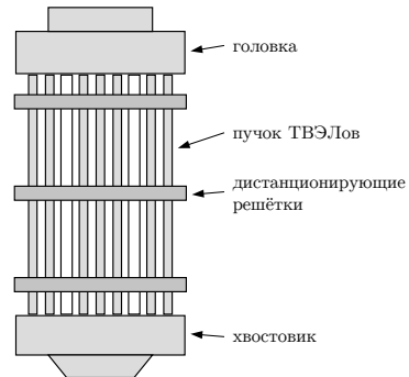
ТВС в сборе
