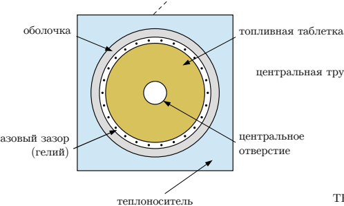
поперечное сечение ТВЭЛа (увеличено)
