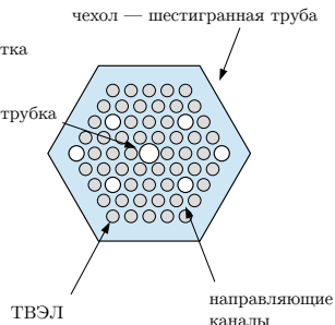
поперечное сечение ТВС
