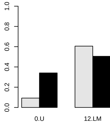
HETARB Mortality
