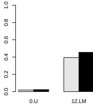
HETARB Topkill-Resprout
