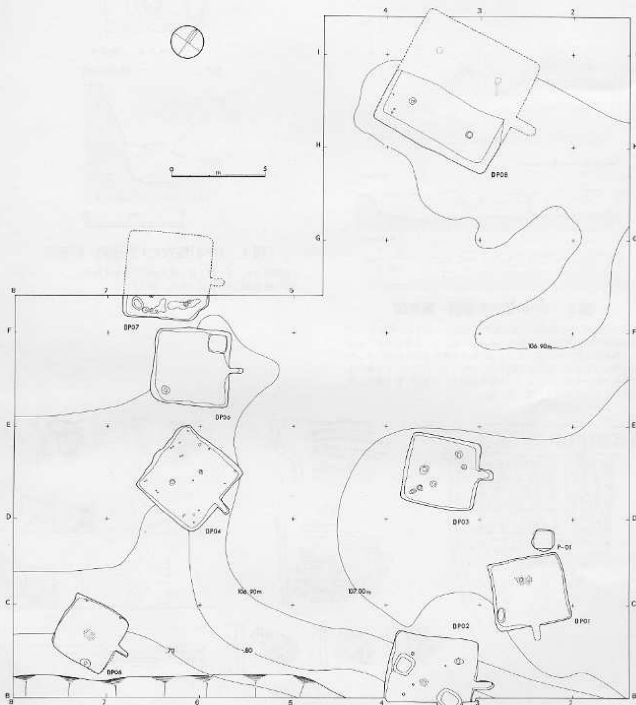
図2 遺構の分布と微地形
