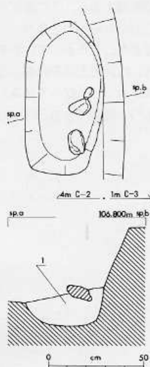
図4 DP01堅穴P1平面図・断面図
