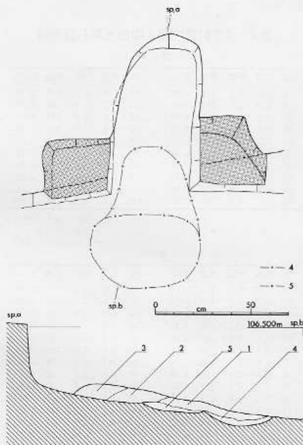
図9 DP 04堅穴カマド平面図・断面図
