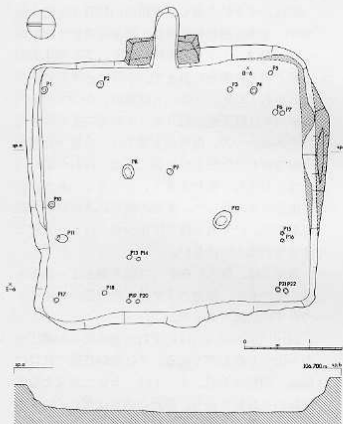
図8 DP 04堅穴平面図・断面図
