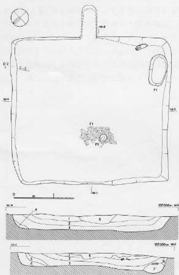
図3 DP01堅穴平面図・断面図
