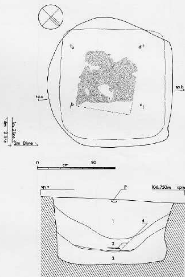
図15 P-01平面図・断面図
