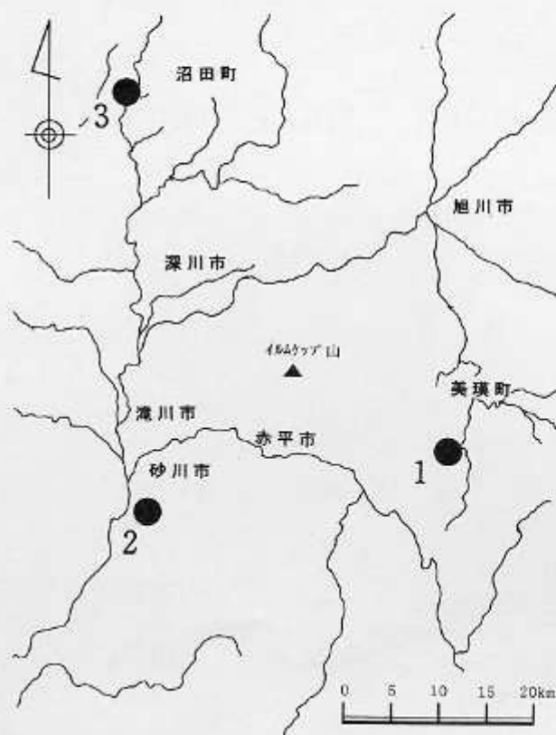
第1図 旭川周辺地域における滝の上動物群の新産地 1. 美瑛, 2. 砂川, 3. 沼田
