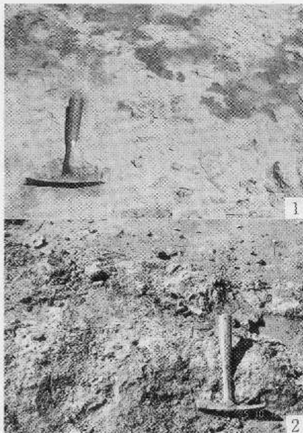
第7図 焼山層の露頭と貝化石包含部
