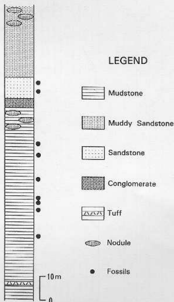
第4図 美開2地点における地質柱状図
