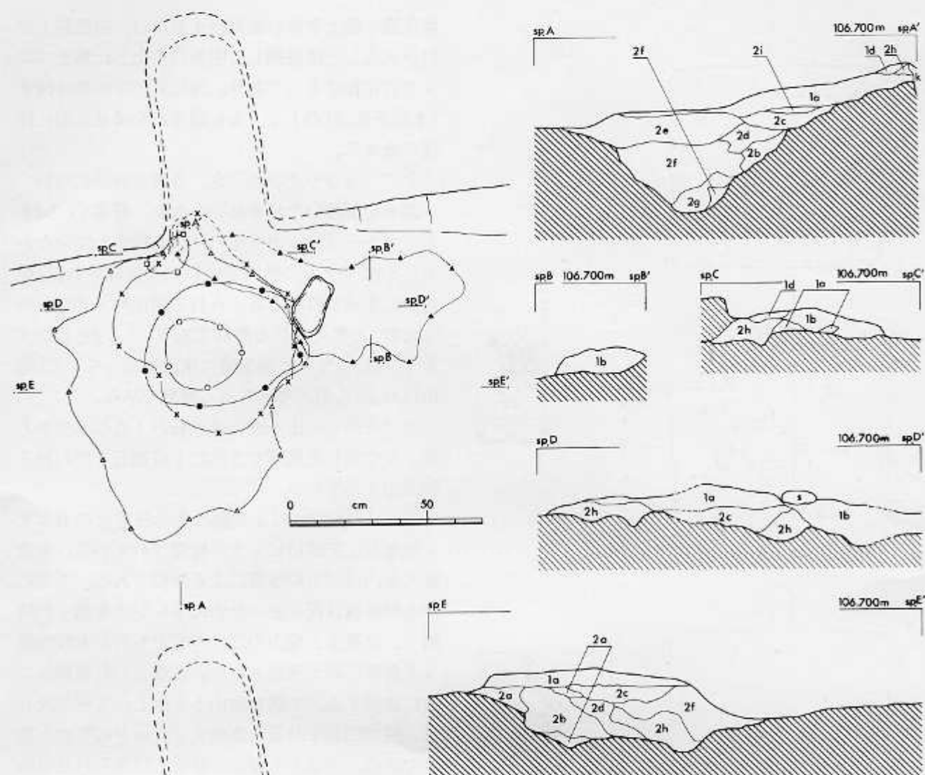
図6 DP01堅穴カマド平面図・断面図
