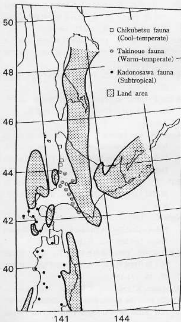
第13図 滝の上動物群、築別動物群および門ノ沢動物群の分布と中期中新世初頭(約16.5~15Ma)における北海道周辺の古地理
