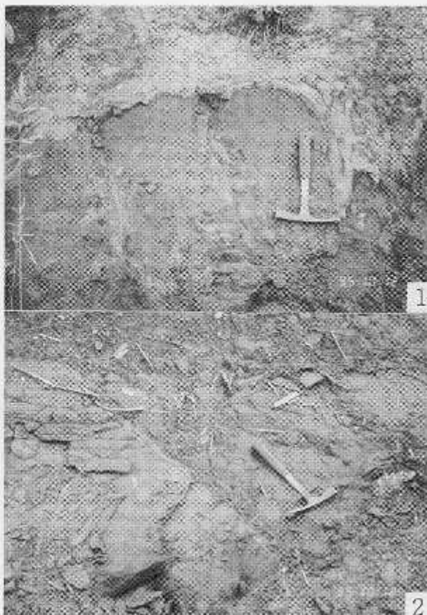
第8図 幌新層の露頭と貝化石包含部
