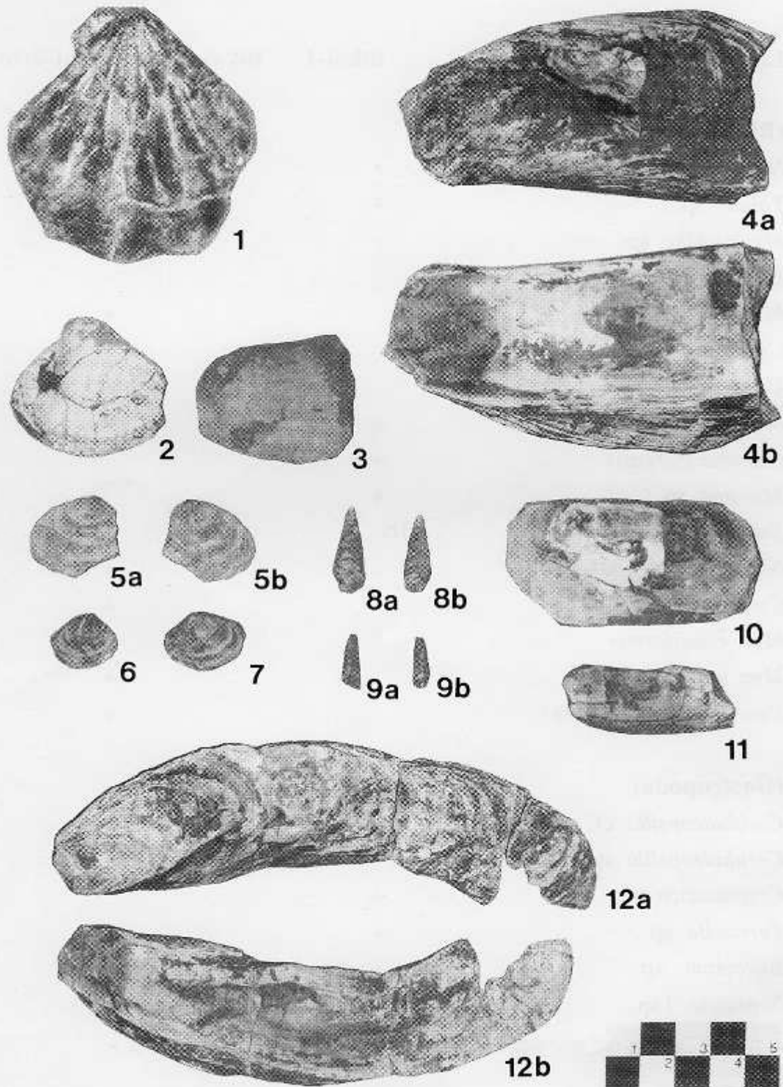
第9図 美開2地点より産出した貝化石
