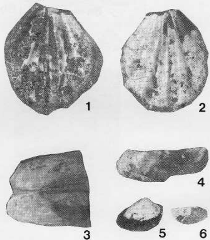
第12図 貝化石群集の古生態学的特徴
