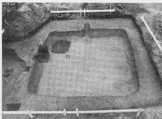
写真12 DP 05堅穴完掘
