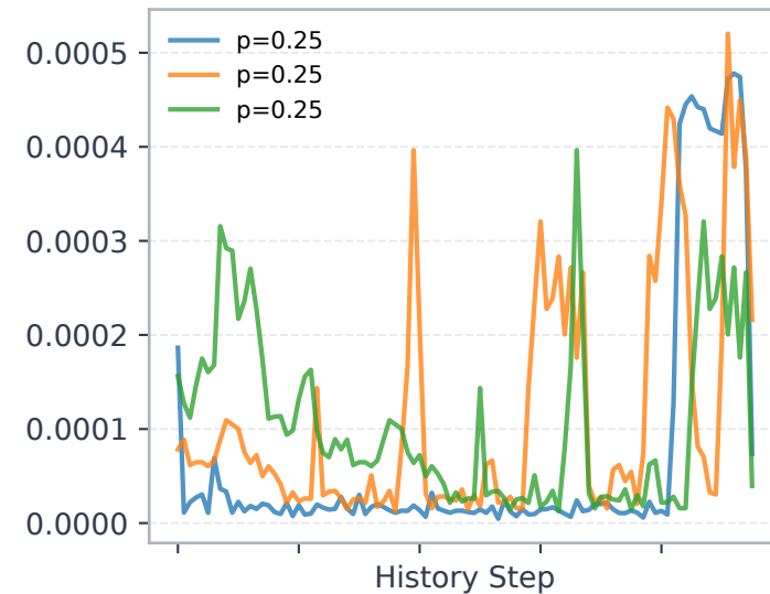
Geant E3
