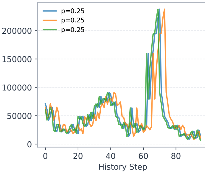
Geant E1
