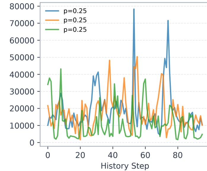
Geant E3
