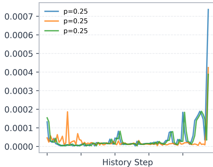
Geant E1
