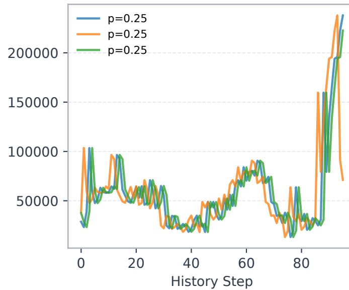
Geant E2
