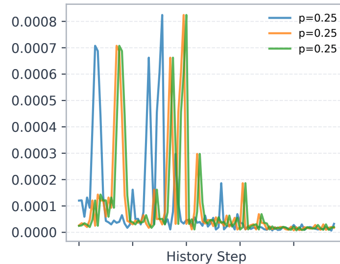
Geant E2
