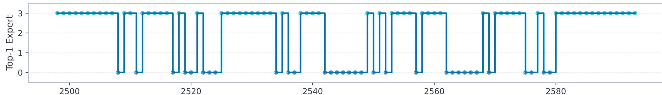
Abilene
