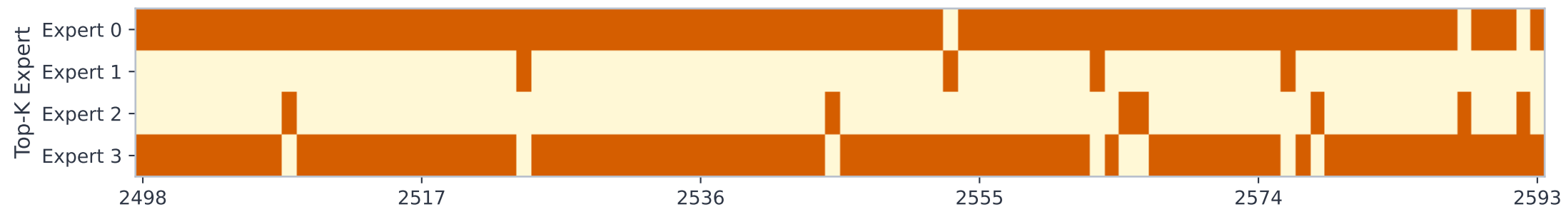
Abilene
