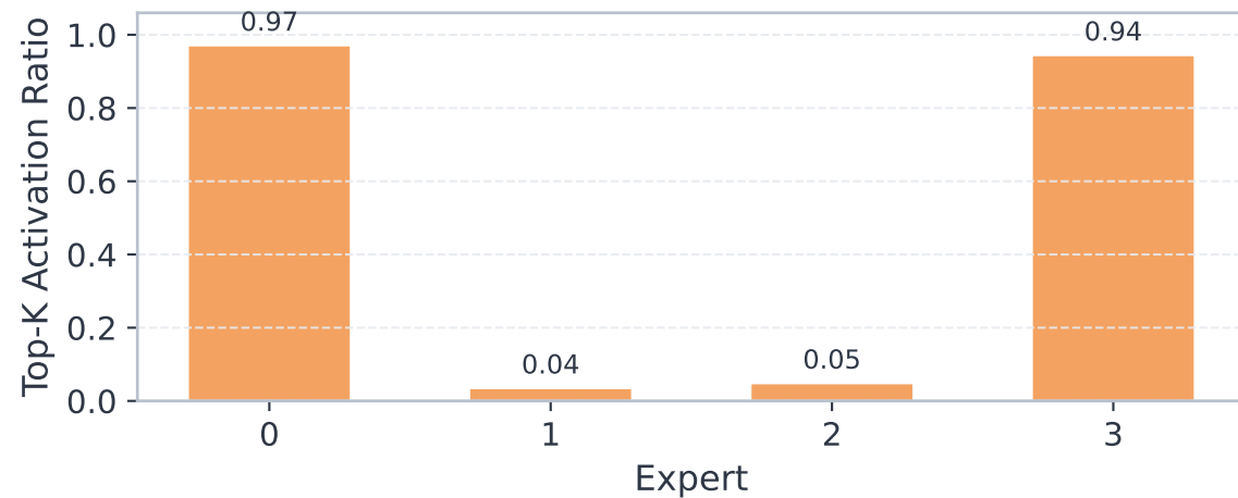
Abilene
