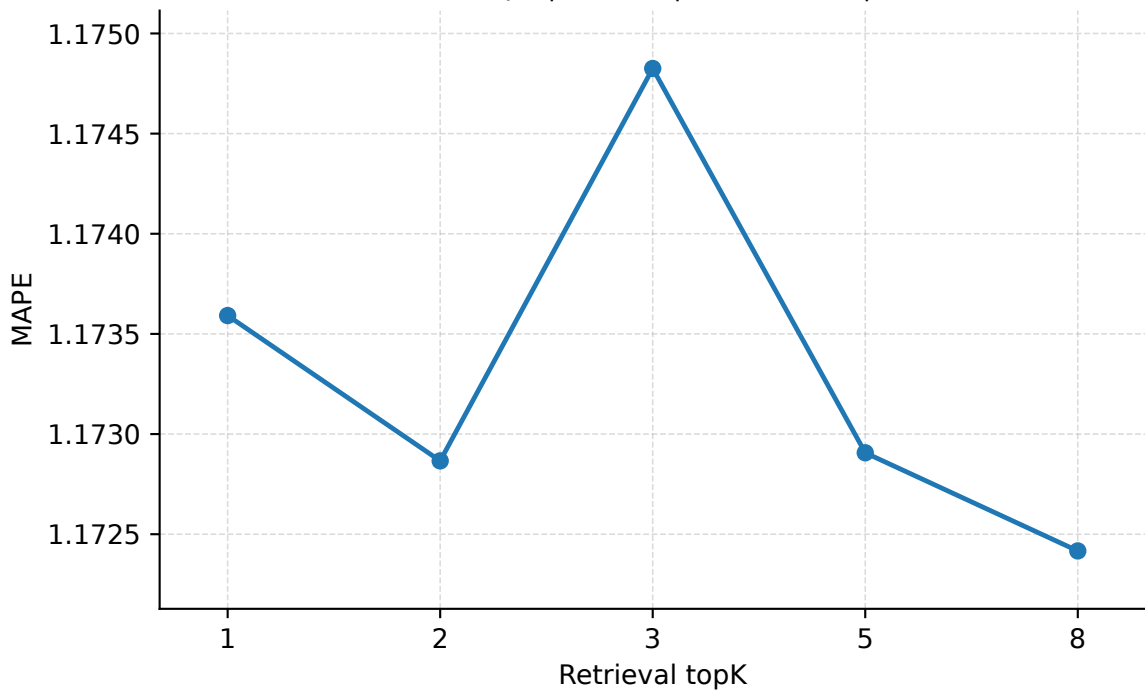
Retrieval topK | Abilene | PredLen=10 | MAPE
