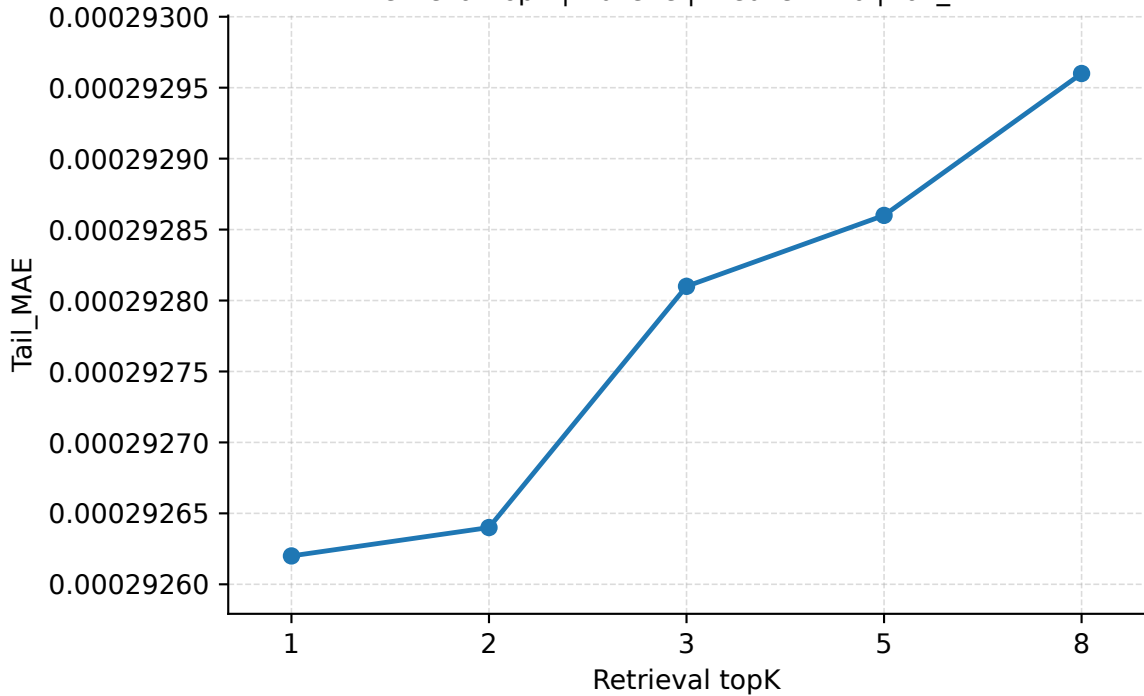
Retrieval topK | Abilene | PredLen=10 | Tail_MAE
