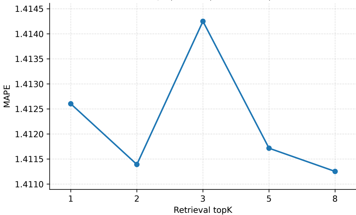
Retrieval topK | Abilene | PredLen=15 | MAPE
