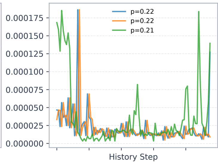
Geant E1
