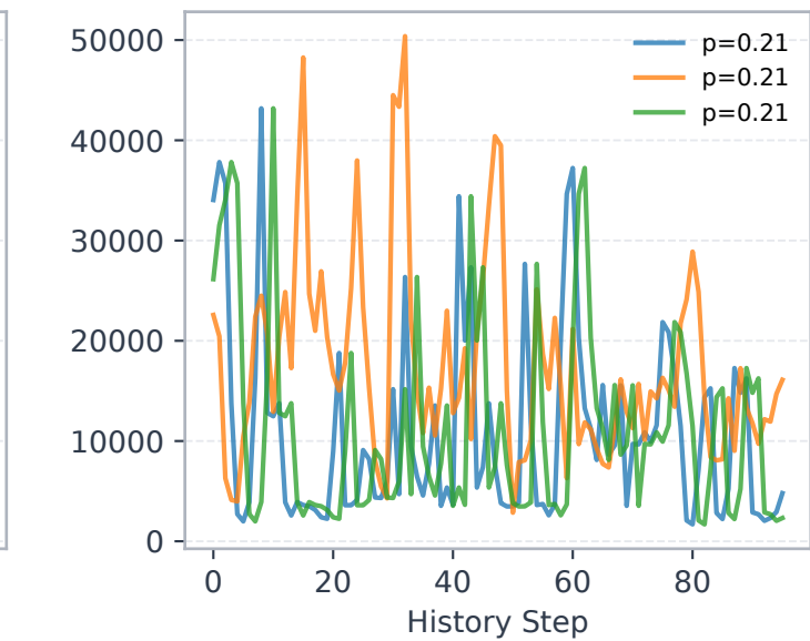
Geant E3
