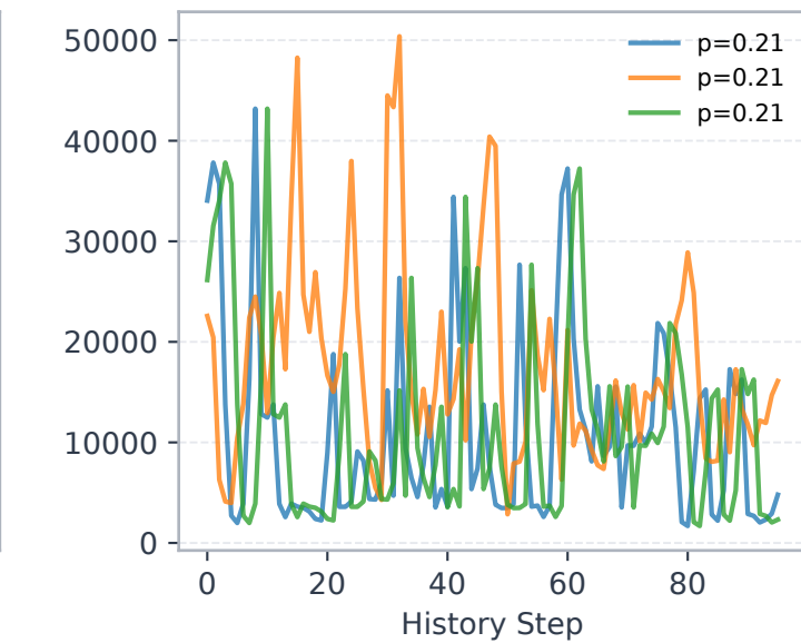
Geant E2
