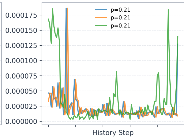
Geant E3
