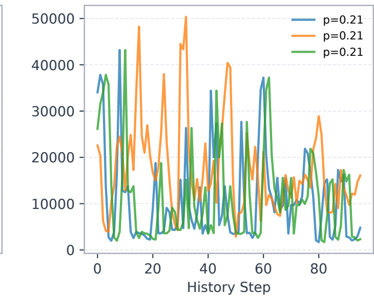
Geant E1
