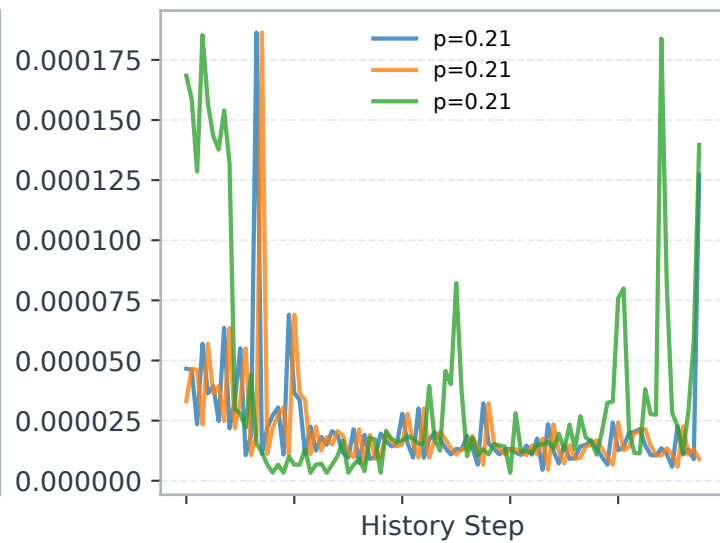
Geant E2
