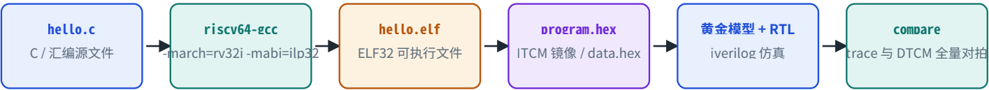
从 C 代码到仿真结果：一条命令里的六个阶段
