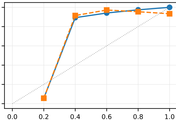
Phi-3.5-mini / GSM8K
