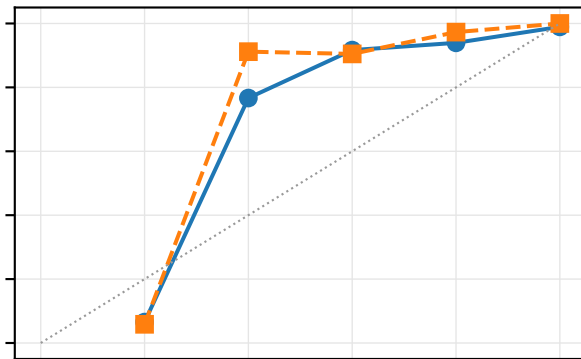
Qwen2.5-3B / GSM8K
