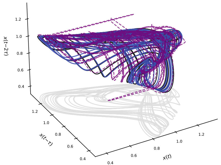
Mackey-Glass ( n = 10 ) (d)
