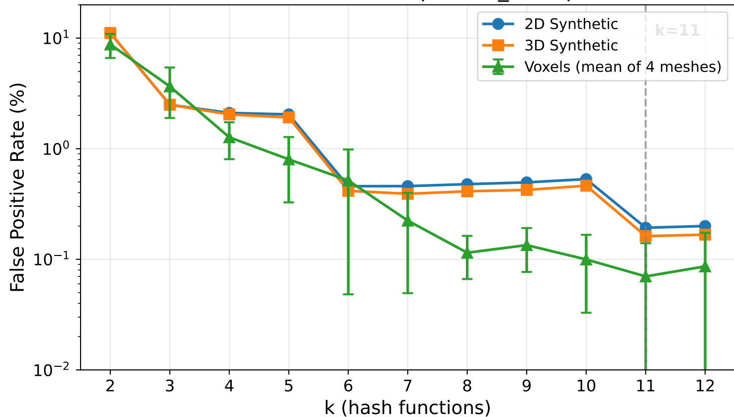
SBBF FPR vs k (Hilbert + pattern_lookup + XOR)
