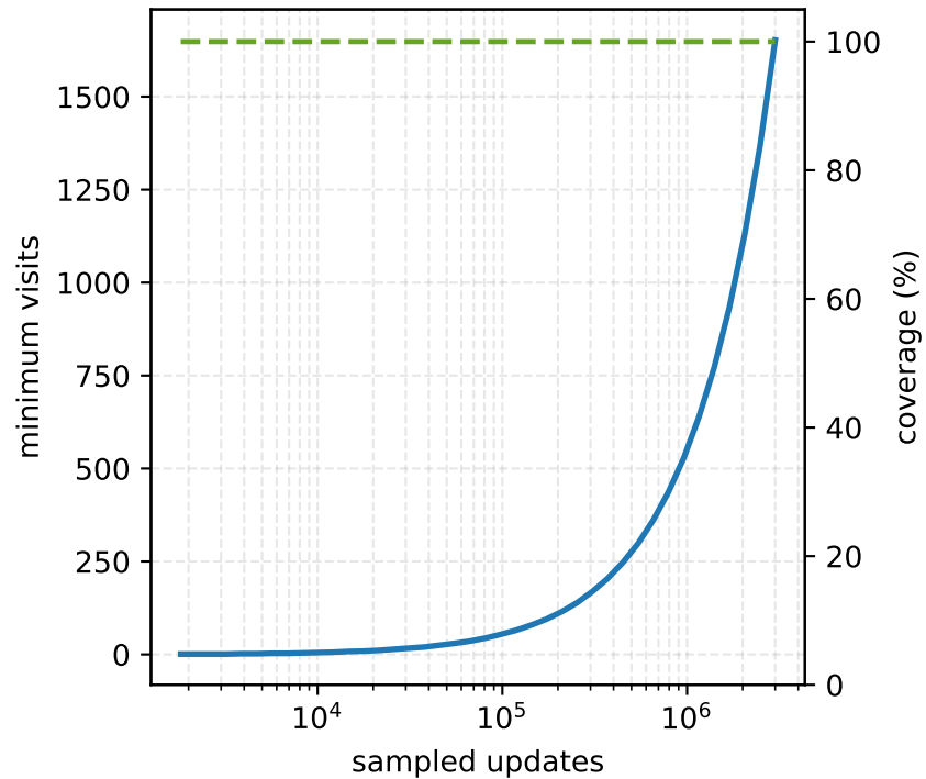
SEIR
