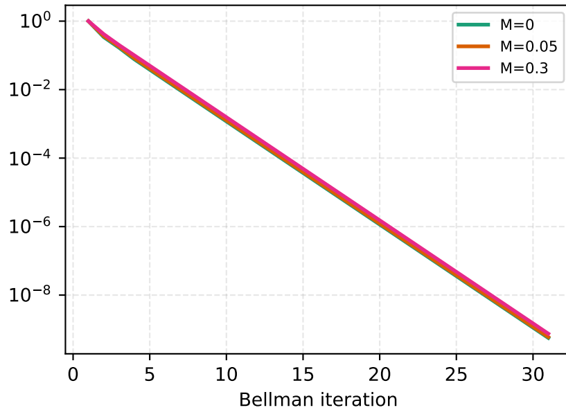
SIS
