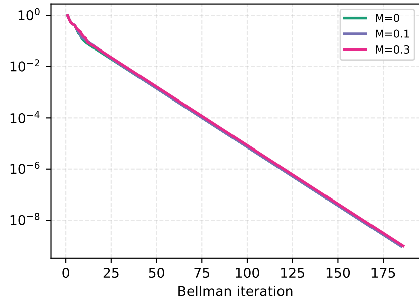
SEIR
